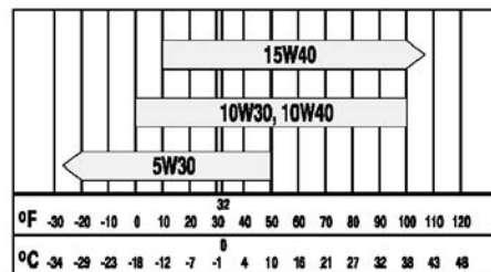
FIGURE 14. VISCOSITÉ DE L'HUILE CONTRE TEMPÉRATURE AMBIANTE
