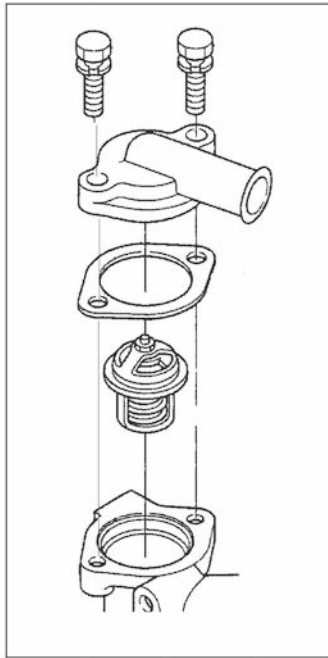
FIGURE 18. THERMOSTAT ET BOÎTIER TYPES
