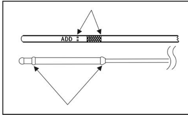
FIGURE 13. REPÈRES ADD/FULL DE LA JAUGE D'HUILE
