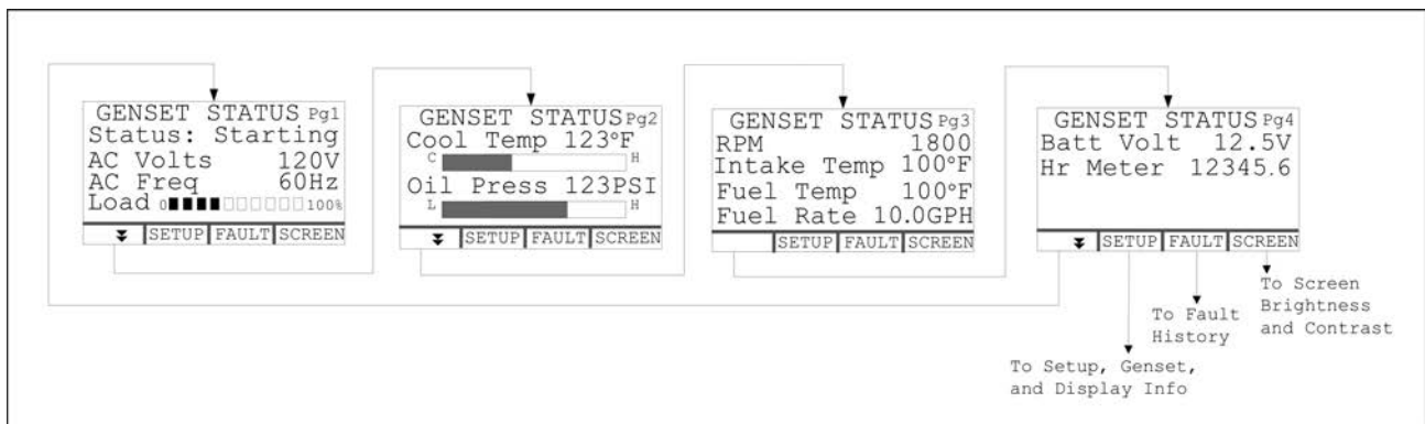
FIGURE 5. ÉCRANS D'ÉTAT DU GROUPE ÉLECTROGÈNE
