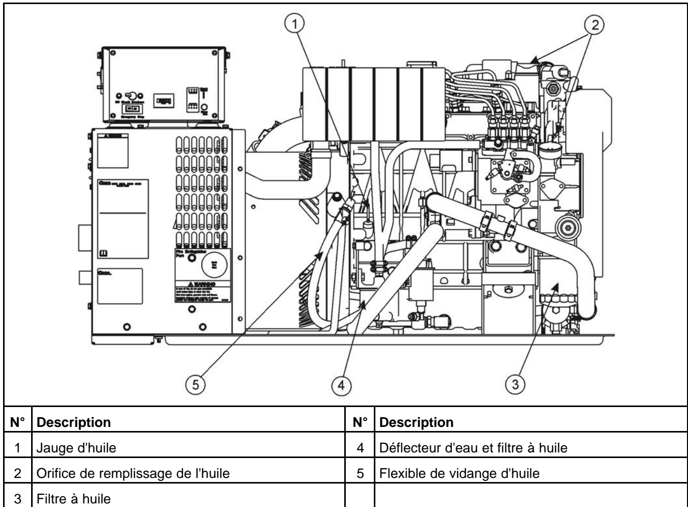
FIGURE 12. POINTS D'ENTRETIEN POUR L'HUILE ET LE CARBURANT
