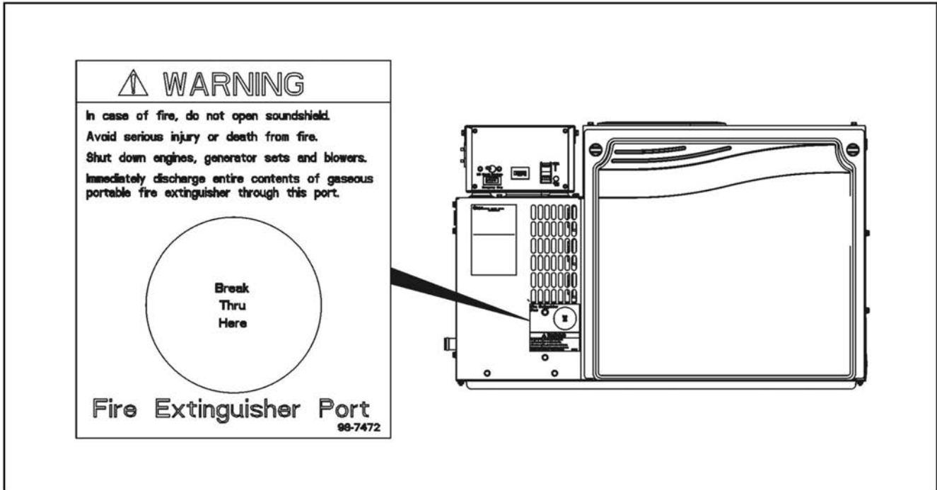
FIGURE 11. EMLACEMENT DE L'ÉTIQUETTE DU PORTE EXTINCTEUR
