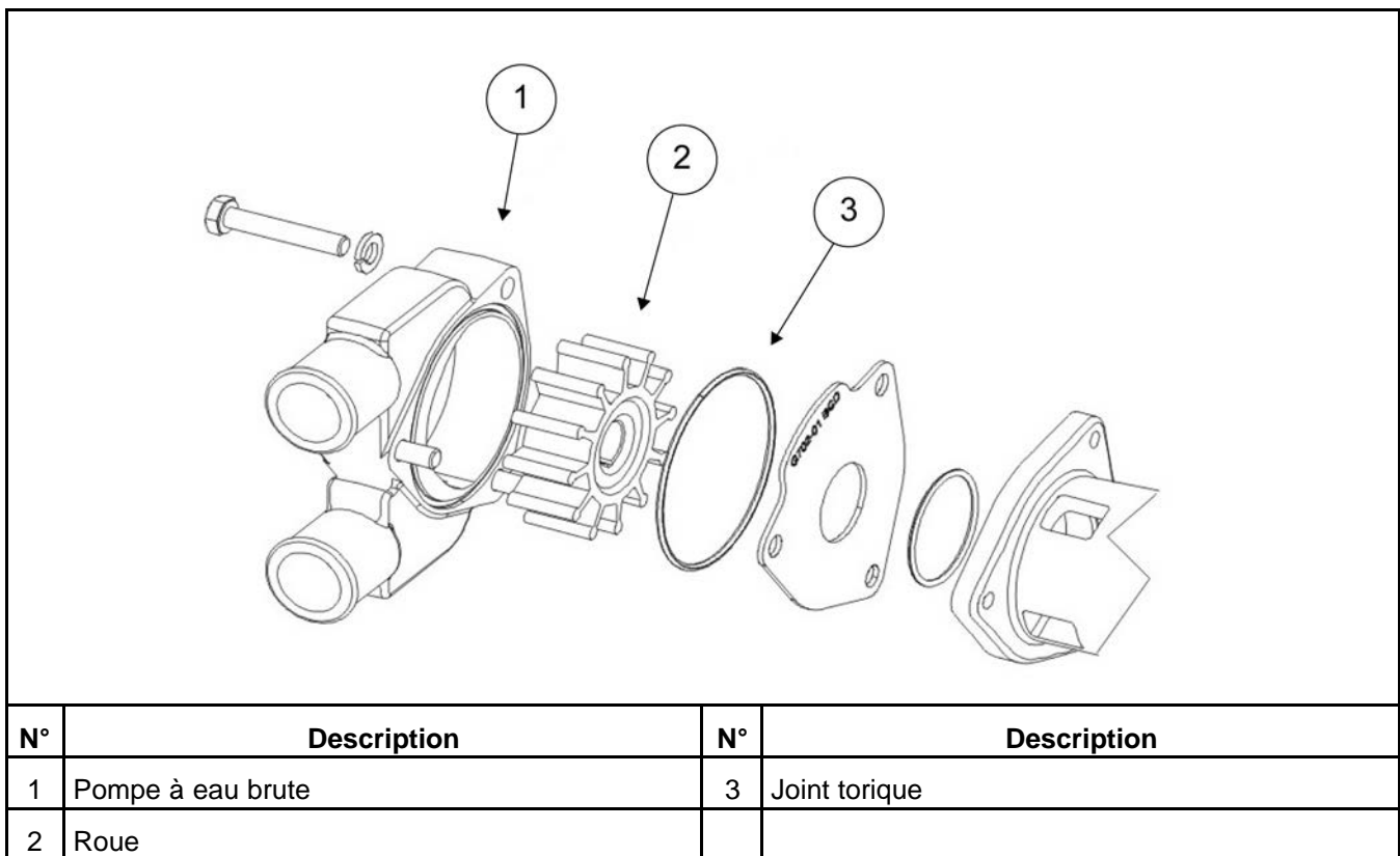
FIGURE 19. REMPLACEMENT DU ROTOR DE LA POMPE À EAU BRUTE
