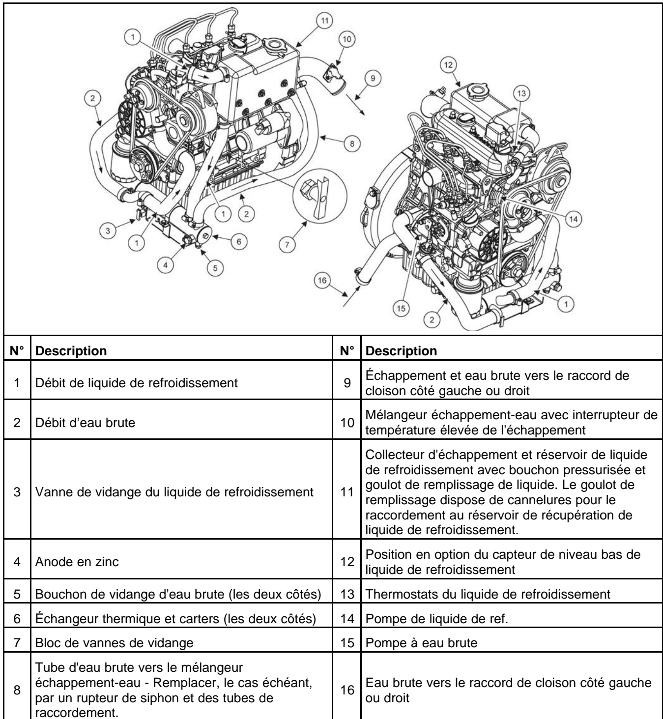
FIGURE 15. COMPOSANTS DU CIRCUIT DE REFROIDISSEMENT
