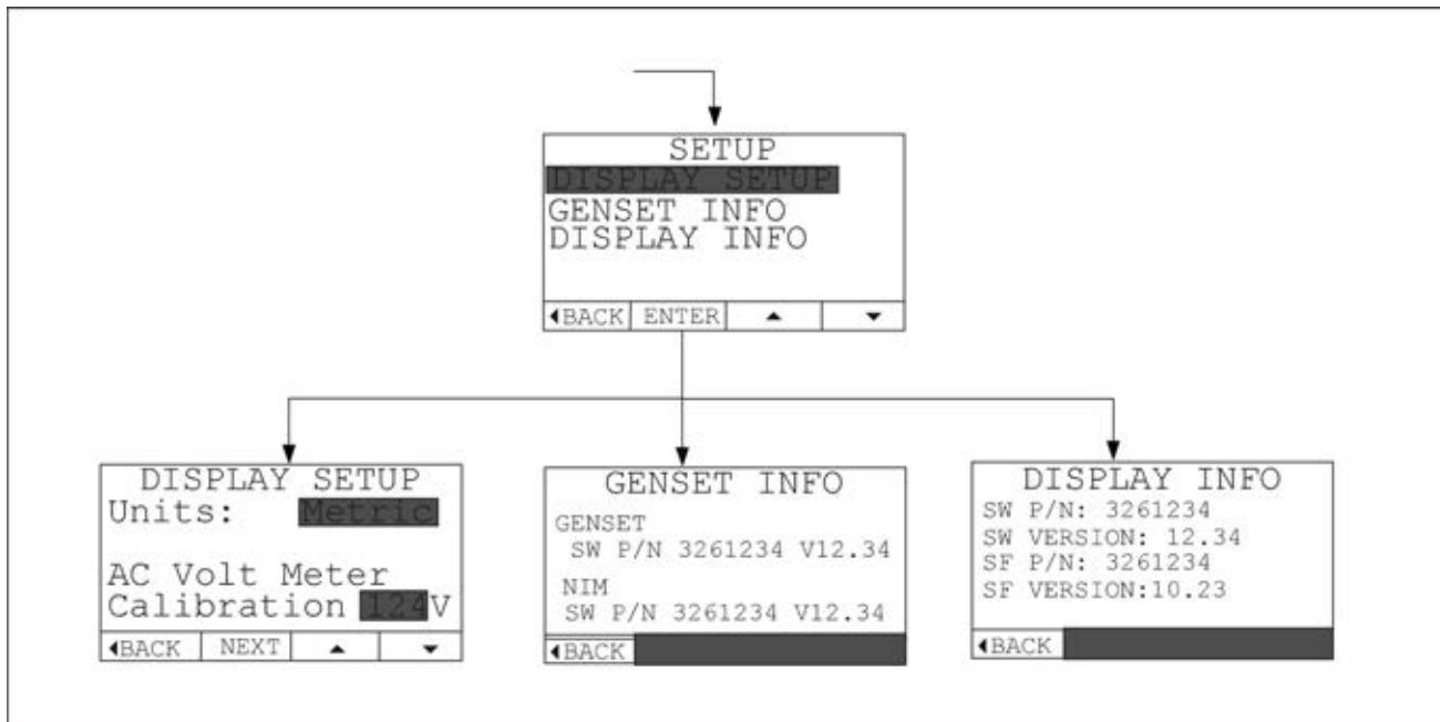
FIGURE 10. CONFIGURATION DE L'AFFICHAGE, INFORMATIONS SUR LE GROUPE ÉLECTROGÈNE ET INFORMATIONS SUR L'AFFICHAGE
