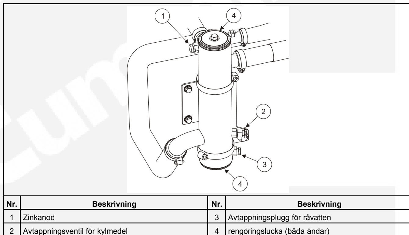
FIGUR 20. VÄRMEVÄXLARE
