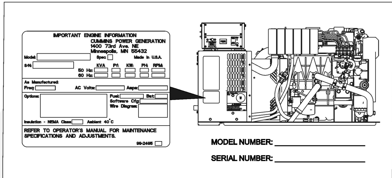
FIGUR 2. NUMMERPLÅTENS PLACERING
