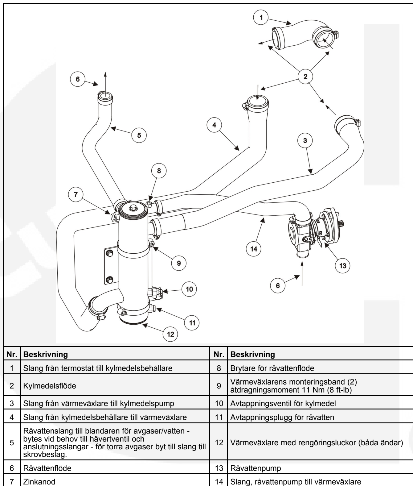
FIGUR 18. MDKDS, MDKDT OCH MDKDU
