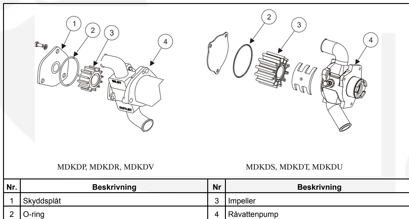
FIGUR 22. BYTE AV RÅVATTENPUMPENS IMPELLER
