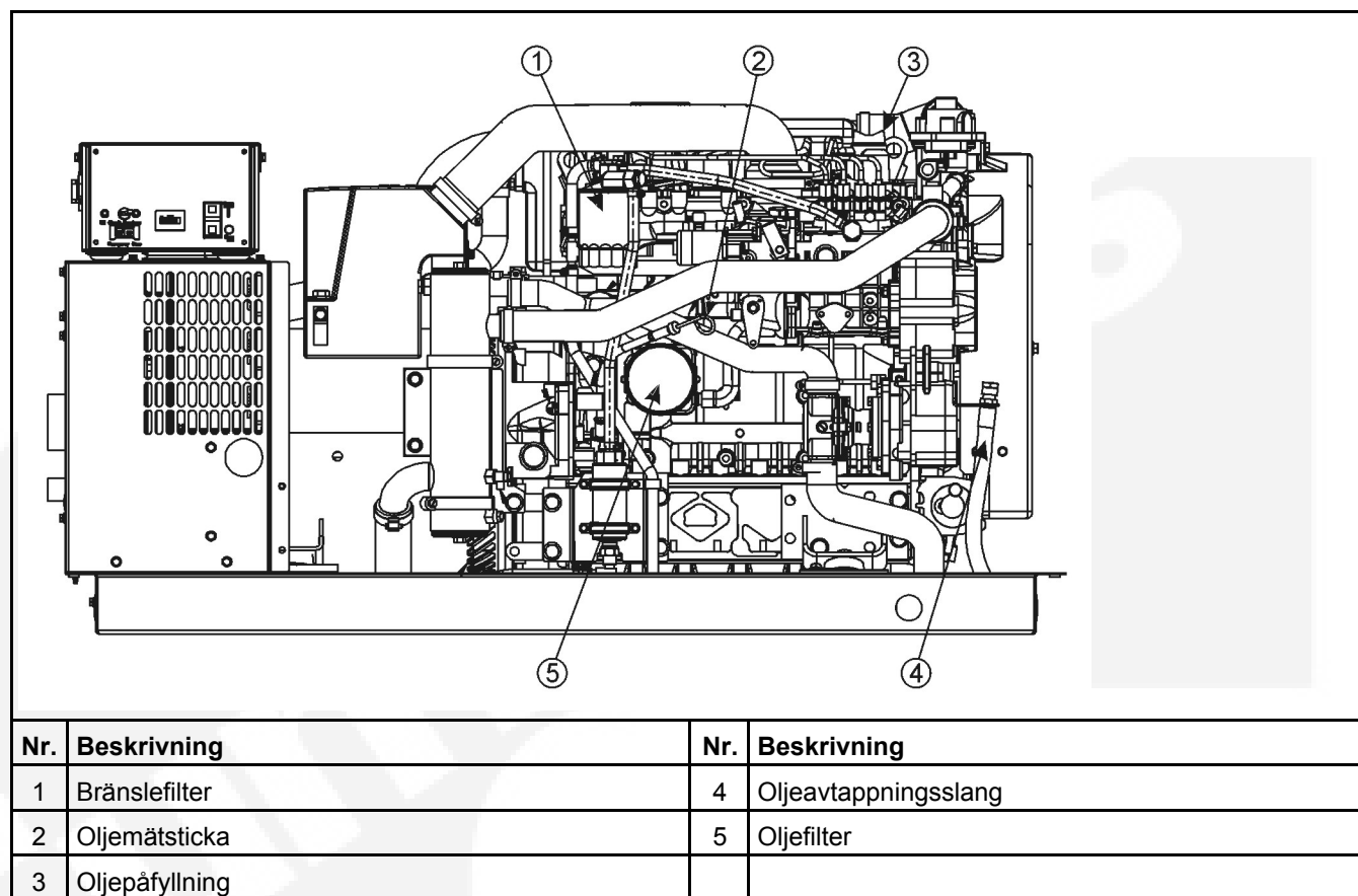
FIGUR 14. SERVICEPUNKTER FÖR OLJA OCH BRÄNSLE - MDKDS, MDKDT OCH MDKDU
