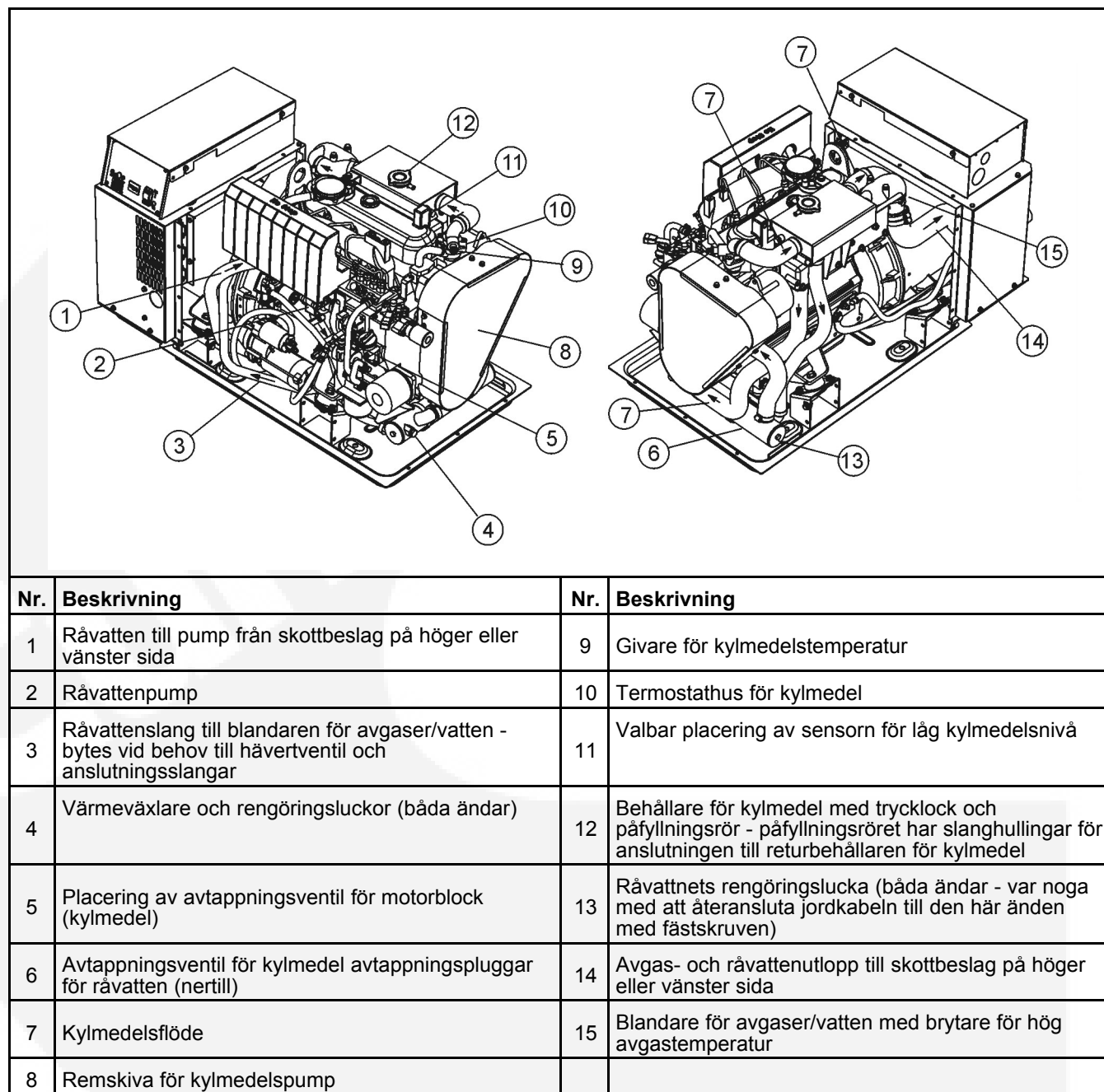
FIGUR 17. MDKDP, MDKDR OCH MDKDV
