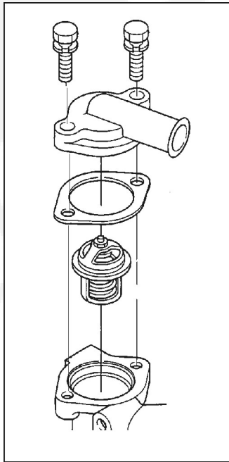
FIGUR 21. TYPISK TERMOSTAT MED HUS
