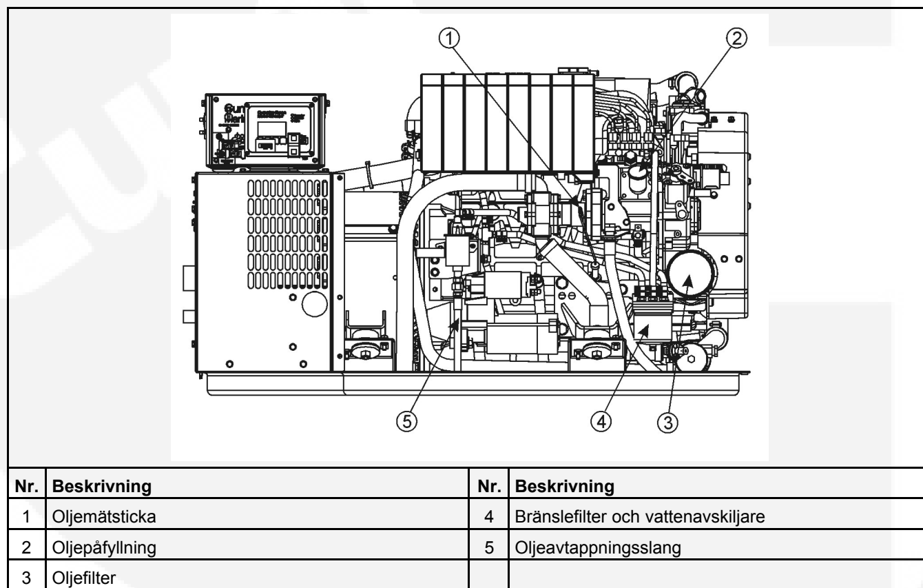
FIGUR 13. SERVICEPUNKTER FÖR OLJA OCH BRÄNSLE - MDKDP, MDKDR, MDKDV
