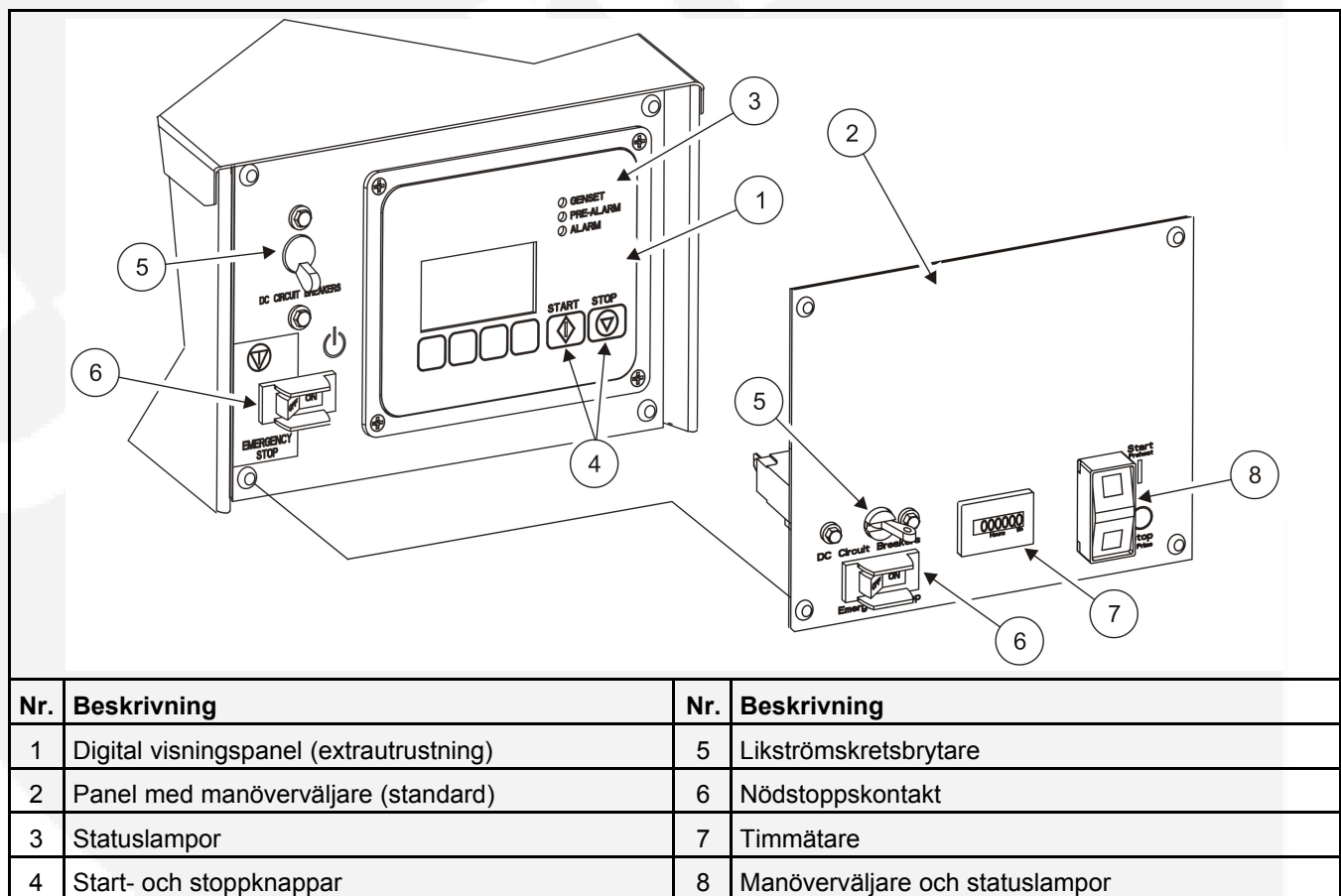
FIGUR 4. KOMPONENTER PÅ GENERATORNS MANÖVERPANEL
