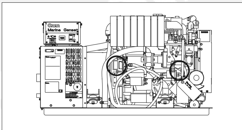
FIGUR 3. TYPISKA PLACERINGAR AV UTSLÄPPSETIKETTER
