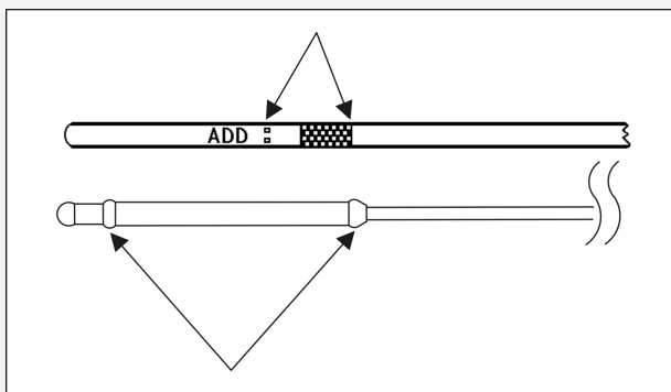
FIGUR 15. MÄTSTICKA FÖR OLJENIVÅ, MARKERINGAR FÖR FYLL/FULL
