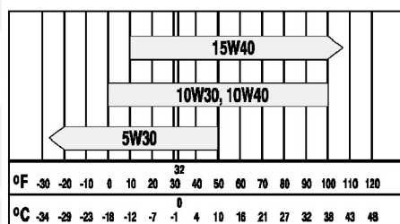
FIGUR 16. OLJEVISKOSITET JÄMFÖRT MED OMGIVANDE TEMPERATUR
