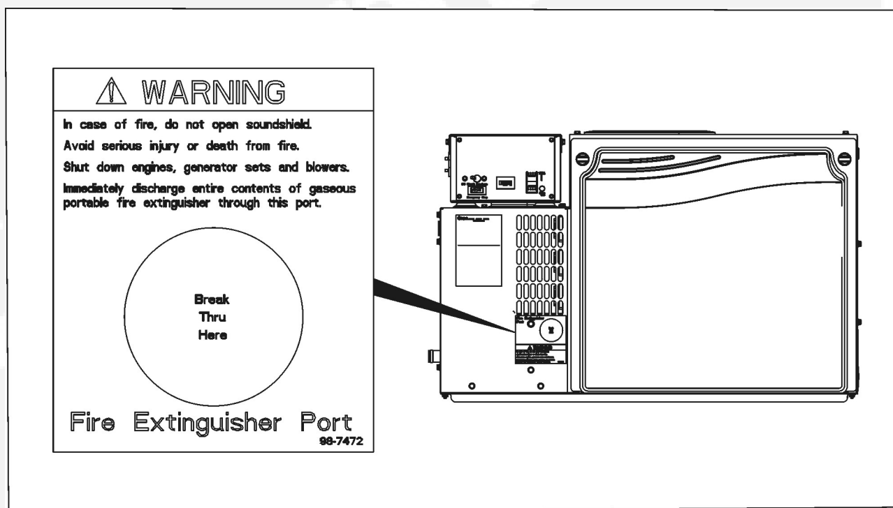
FIGURA 12. POSIZIONE DELL'ETICHETTA SULLA PORTA ESTINTORE
