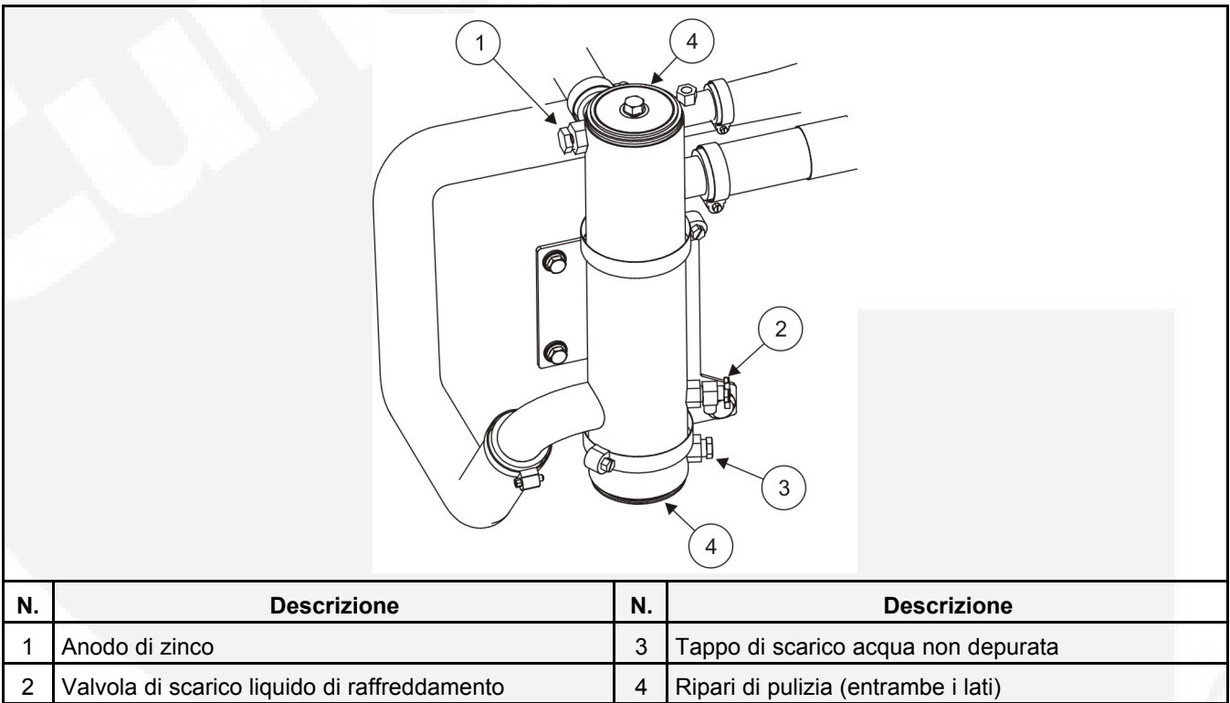
FIGURA 20. SCAMBIATORE DI CALORE
