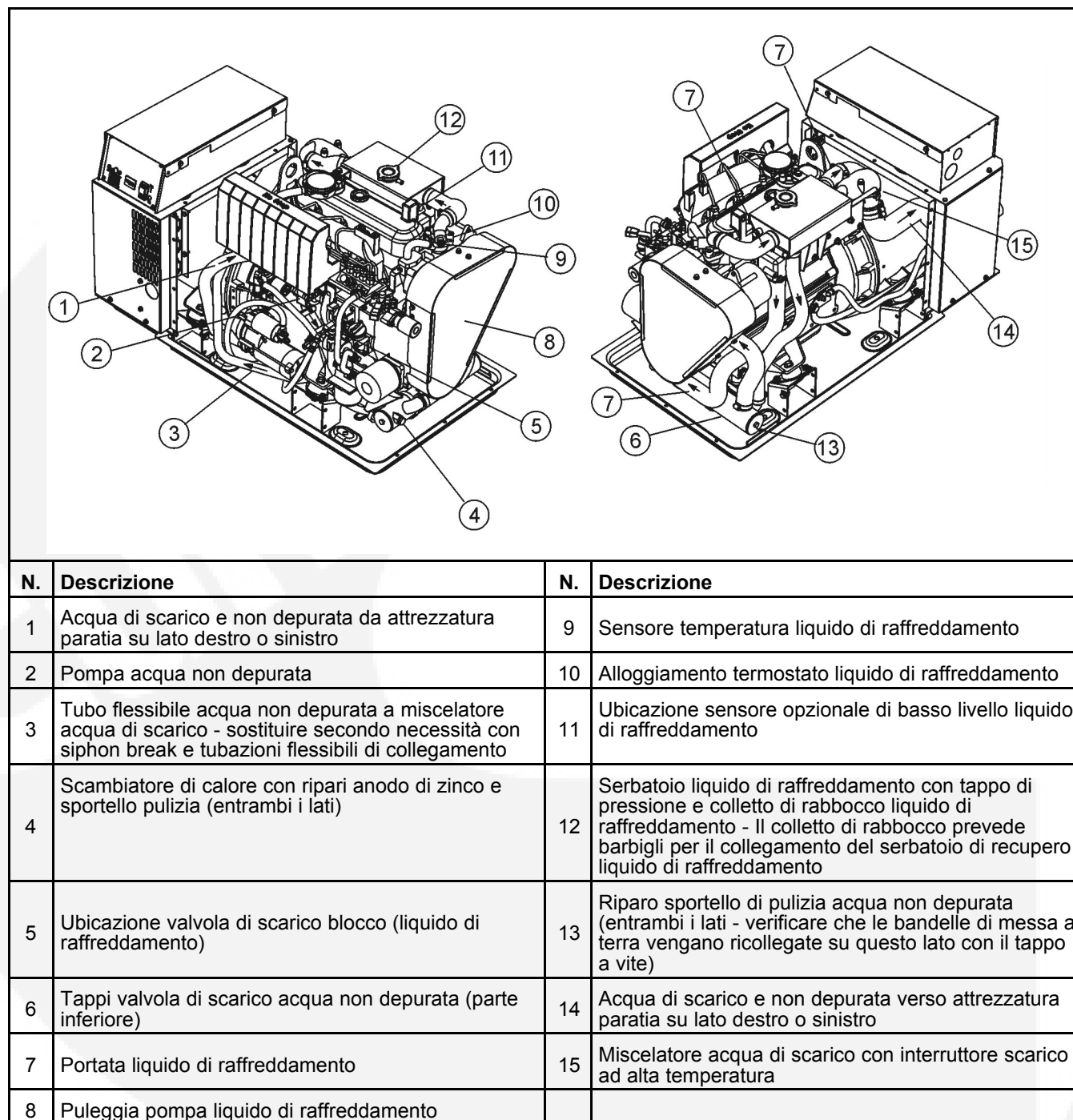
FIGURA 17. MDKDP, MDKDR E MDKDV
