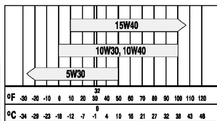
FIGURA 16. VISCOSITÀ DELL'OLIO IN FUNZIONE DELLA TEMPERATURA AMBIENTE
