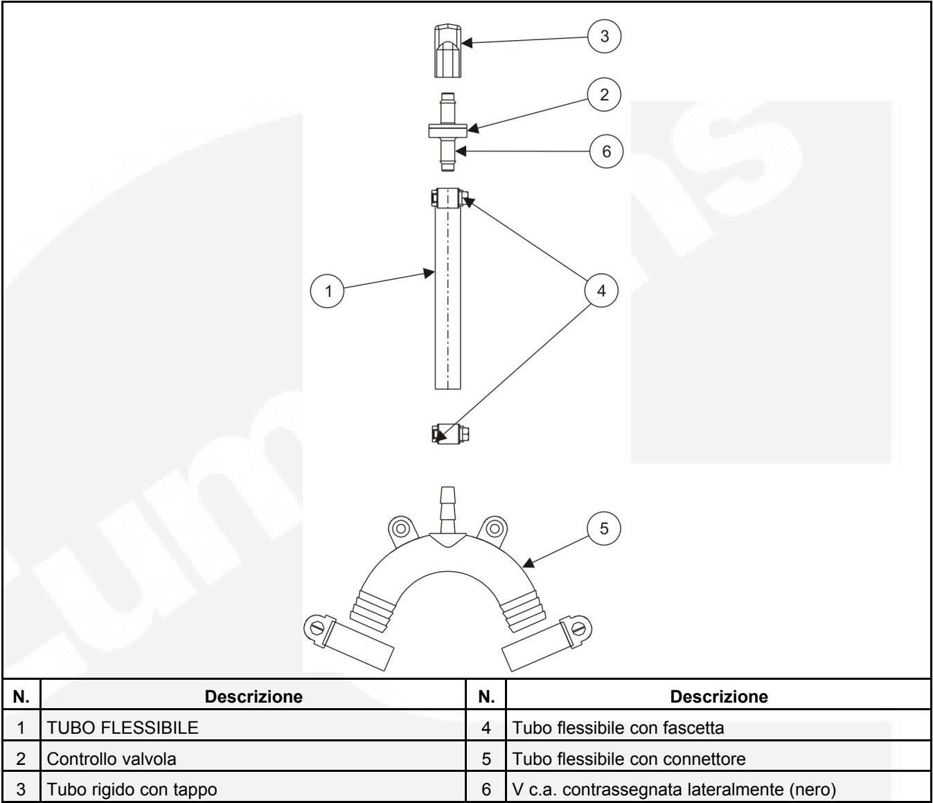
FIGURA 19. GIUNTO A SIFONE
