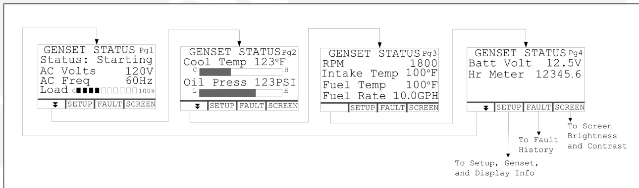
FIGURA 6. SCHERMATE DI STATO DEL GRUPPO GENERATORE
