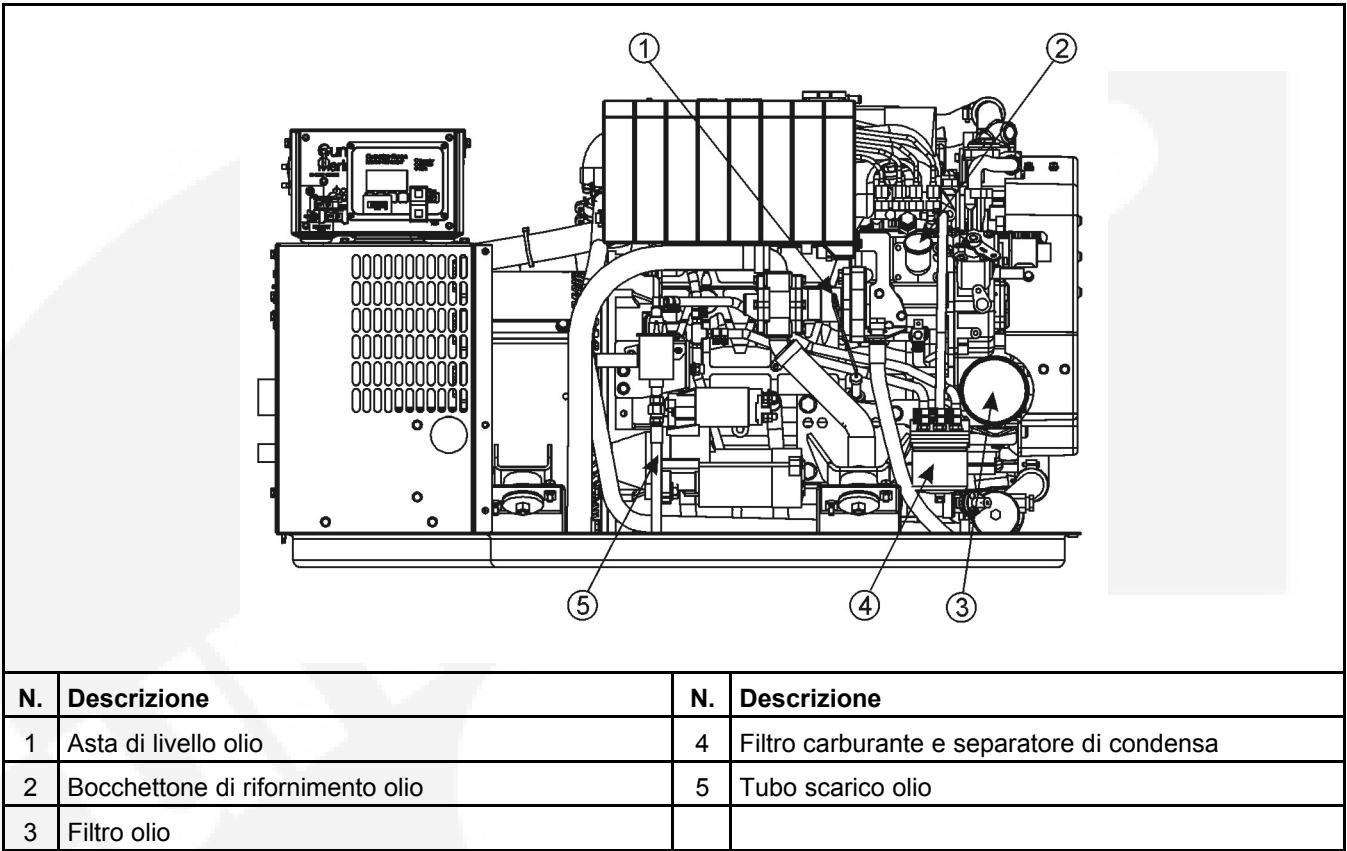
FIGURA 13. PUNTI DI RABBOCCO OLIO E CARBURANTE: MDKDP, MDKDR, MDKDV
