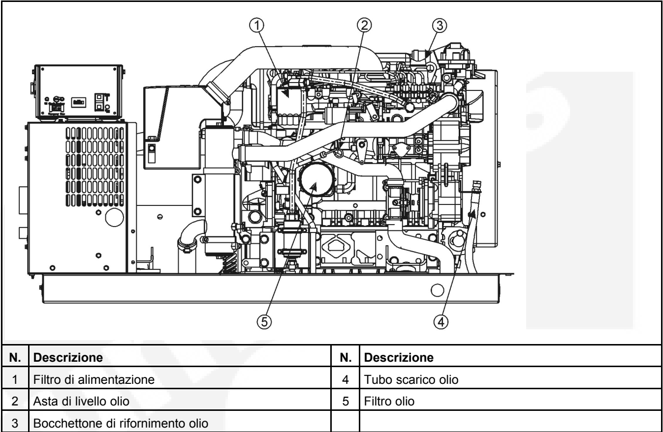
FIGURA 14. PUNTI DI RABBOCCO OLIO E CARBURANTE: MDKDS, MDKDT E MDKDU
