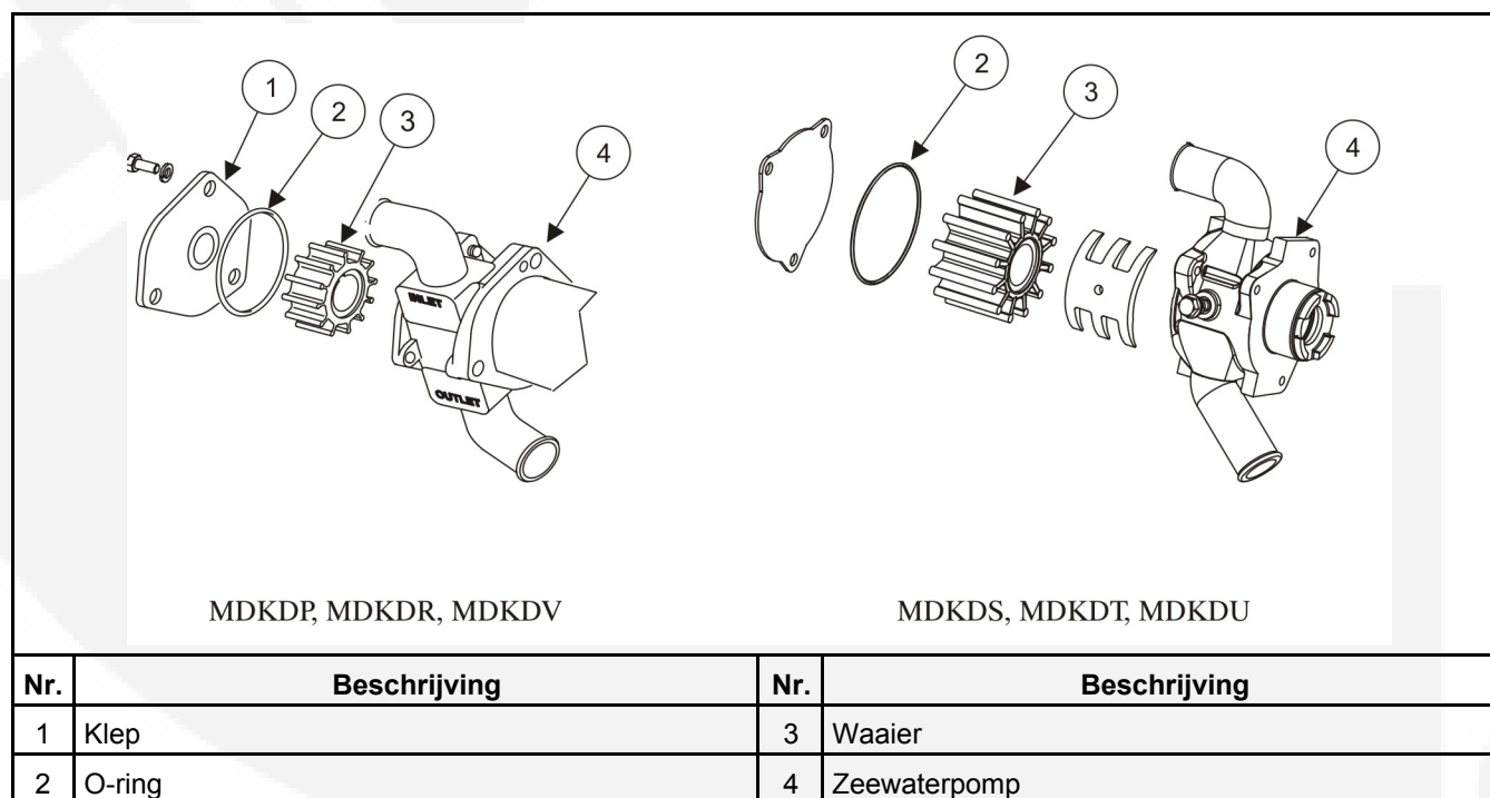
AFBEELDING 22. POMPWAAIER VAN ZEEWATERPOMP VERVANGEN
