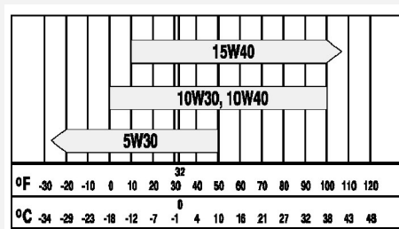
AFBEELDING 16. OLIEVISCOSITEIT VERSUS OMGEVINGSTEMPERATUUR
