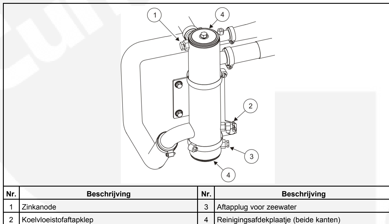
AFBEELDING 20. WARMTEWISSELAAR
