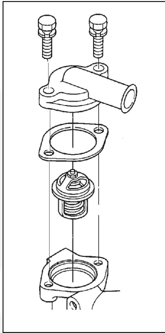
AFBEELDING 21. TYPISCHE THERMOSTAAT MET HUIS
