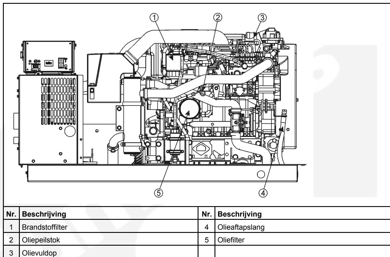
AFBEELDING 14. SERVICEPUNTEN VOOR OLIE EN BRANDSTOF - MDKBT, MDKBU
