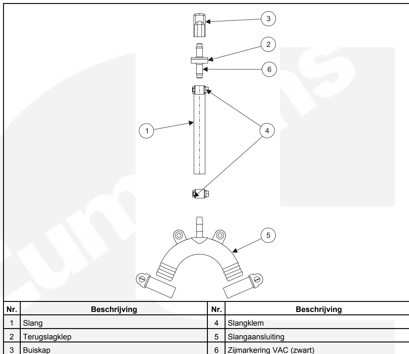
AFBEELDING 19. SIFONONDERBREKING
