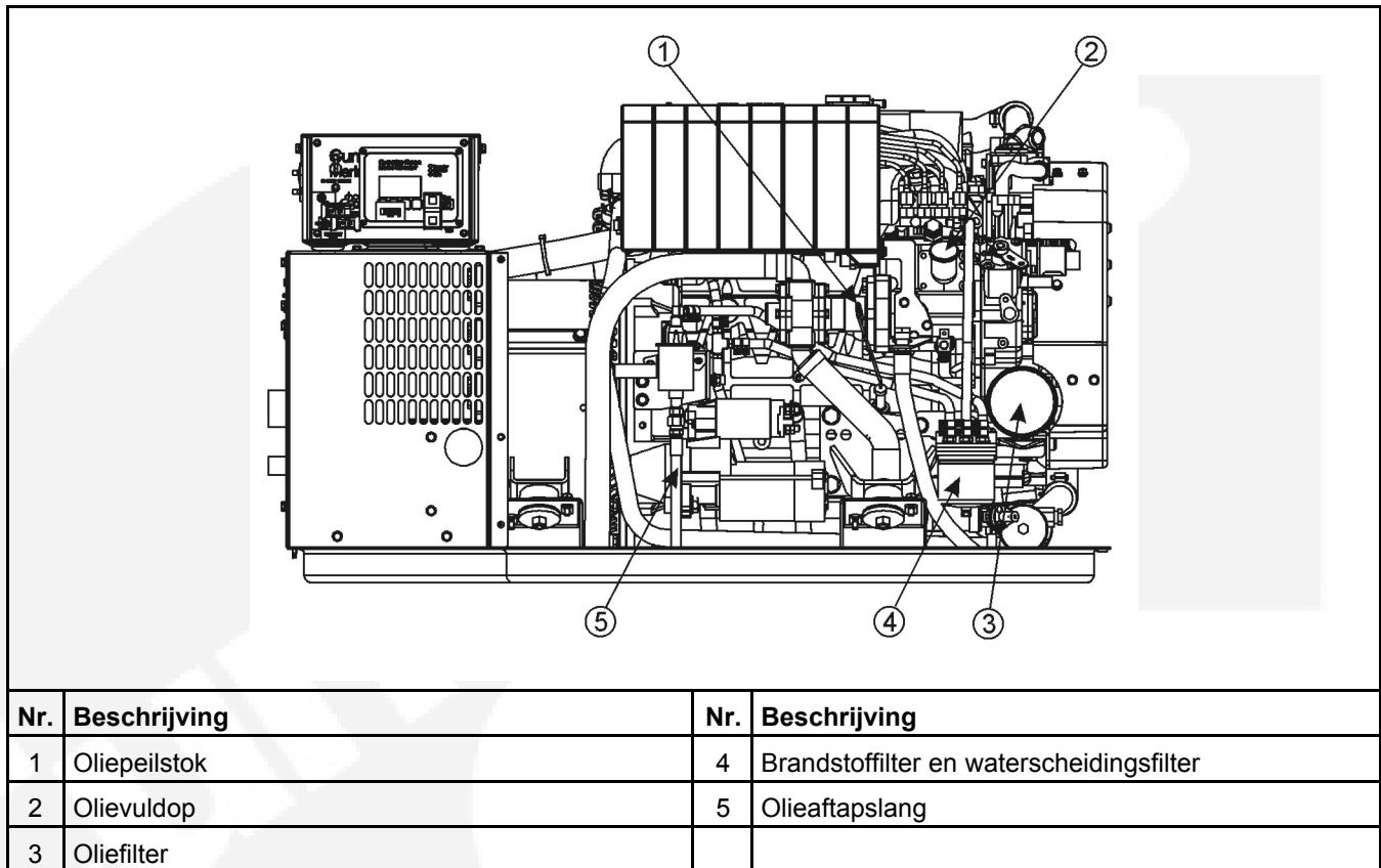
AFBEELDING 13. SERVICEPUNTEN VOOR OLIE EN BRANDSTOF - MDKBP, MDKBR, MDKBV
