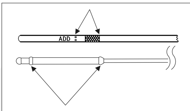
FIGURE 14. REPÈRES ADD/FULL DE LA JAUGE D'HUILE
