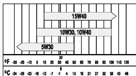
FIGURE 15. VISCOSITÉ DE L'HUILE CONTRE TEMPÉRATURE AMBIANTE
