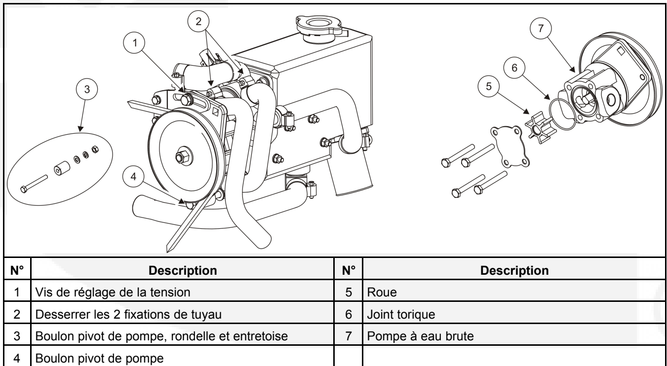
FIGURE 20. DÉPOSE DE LA POMPE À EAU BRUTE
