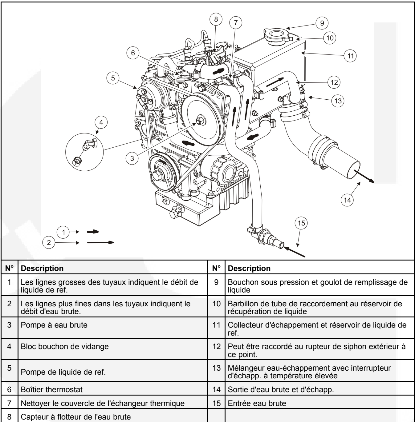
FIGURE 16. CIRCUIT DE REFROIDISSEMENT
