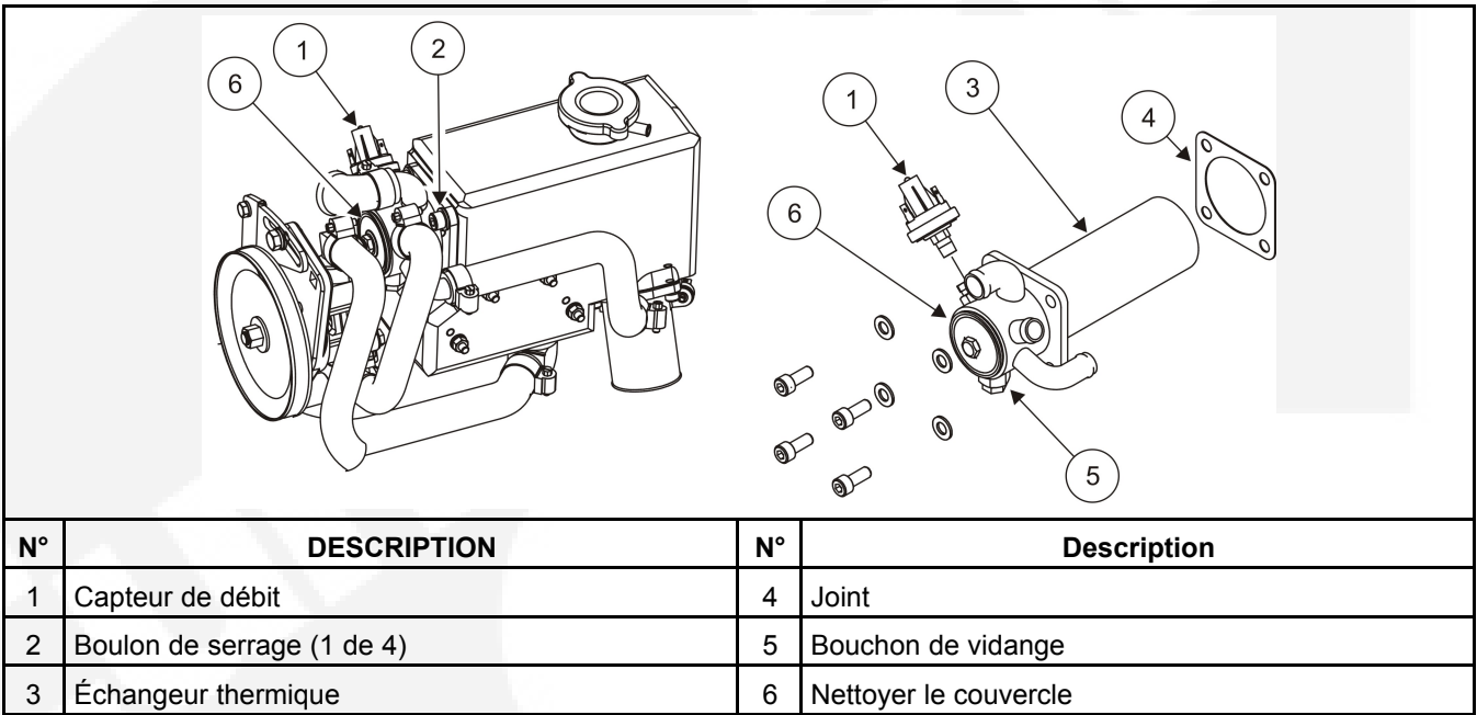
FIGURE 18. ÉCHANGEUR THERMIQUE
