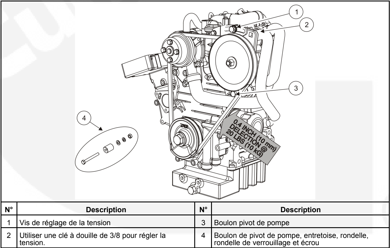
FIGURE 21. RÉGLAGE DE LA TENSION DE LA COURROIE TRAPÉZOÏDALE
