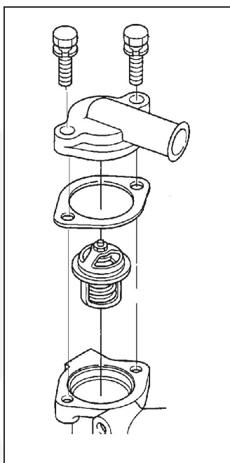
FIGURE 19. THERMOSTAT ET BOÎTIER TYPES
