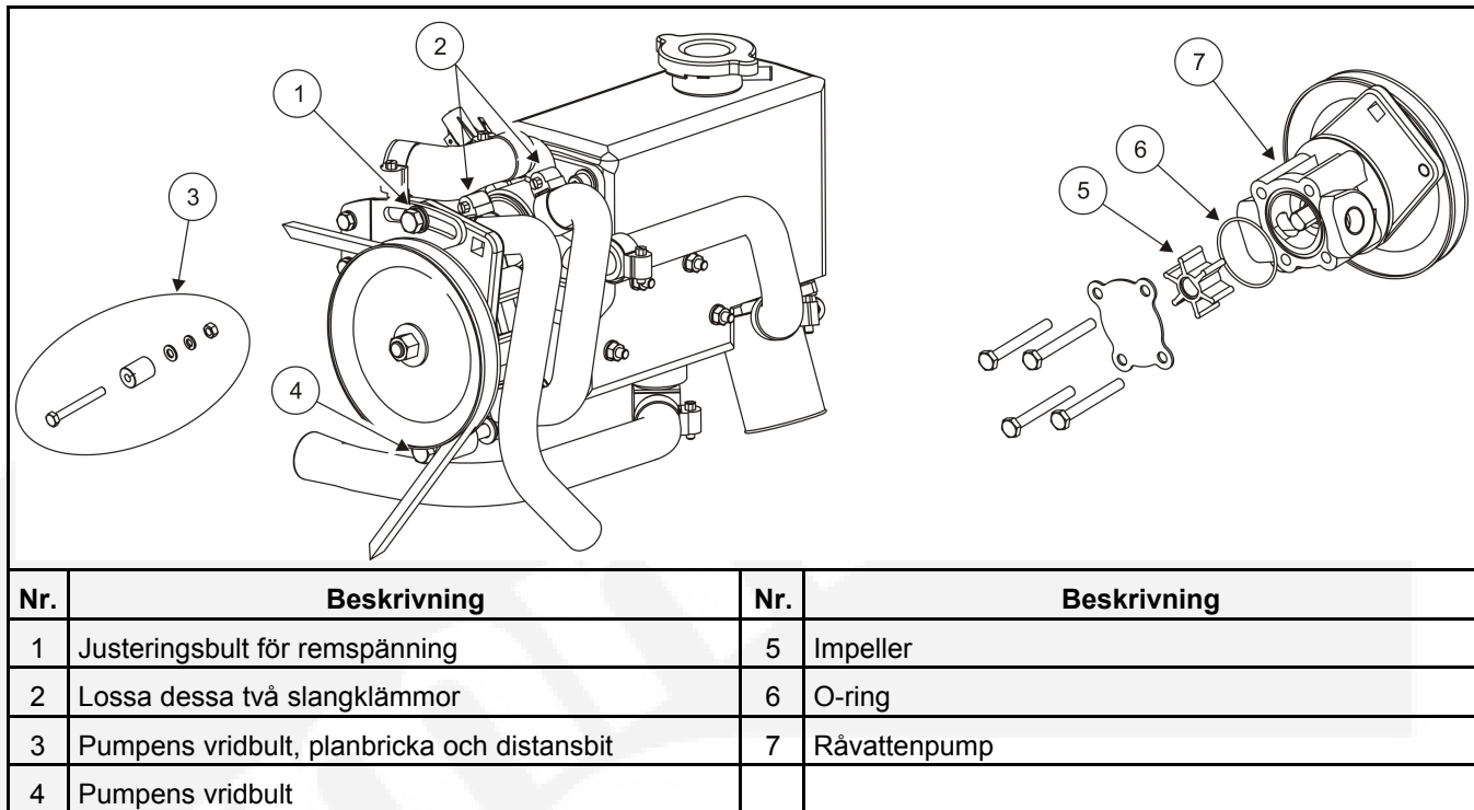
FIGUR 20. BORTTAGNING AV RÅVATTENPUMP
