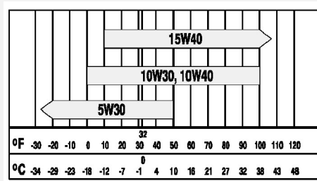
FIGUR 15. OLJEVISKOSITET JÄMFÖRT MED OMGIVANDE TEMPERATUR
