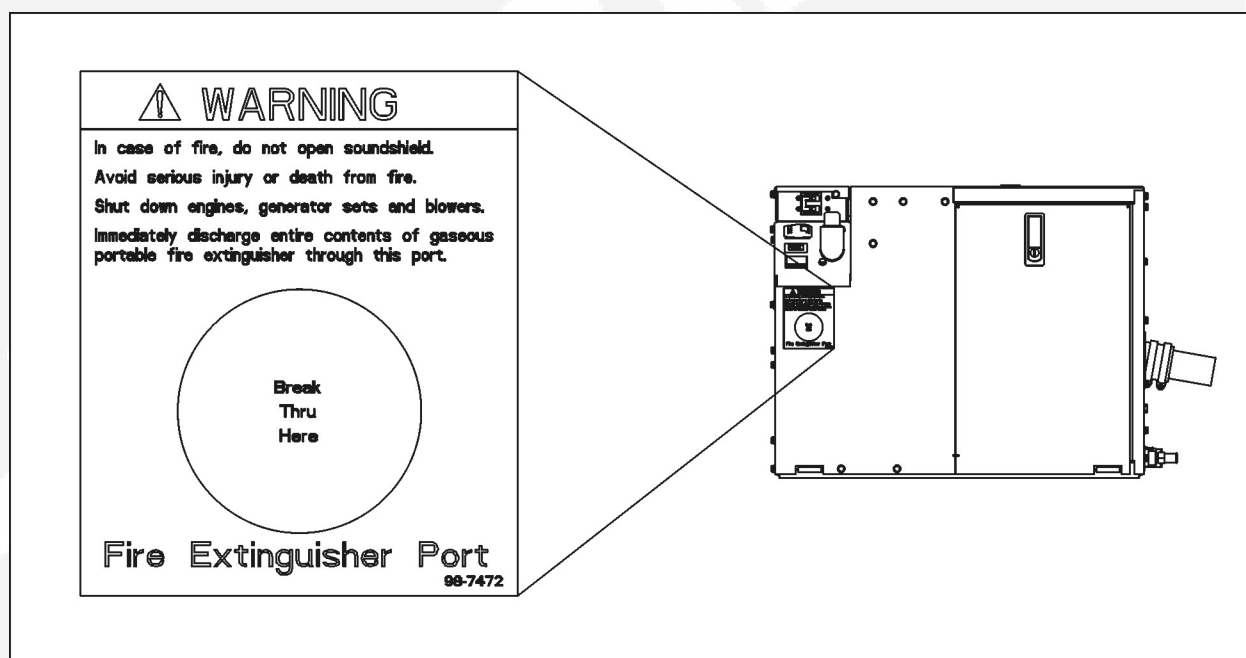
FIGUR 12. PLACERING FÖR ELDSLÄCKARÖPPNINGENS SKYLTT
