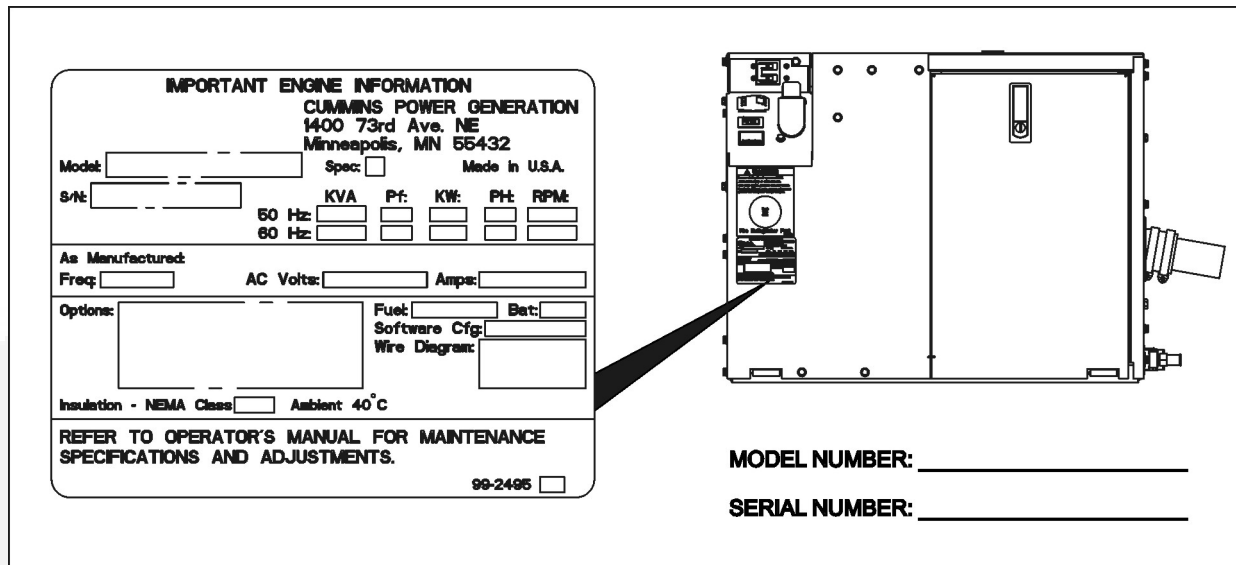
FIGUR 2. NUMMERPLÅTENS PLACERING
