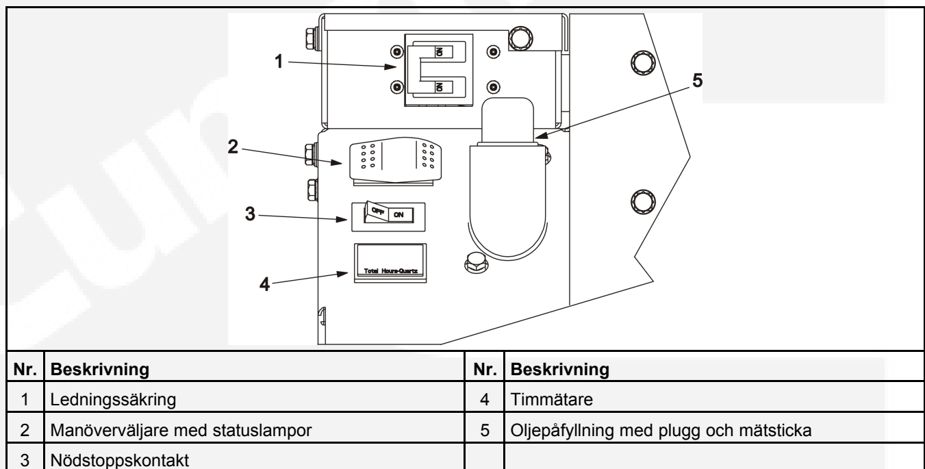
FIGUR 4. KOMPONENTER PÅ GENERATORNS MANÖVERPANEL
