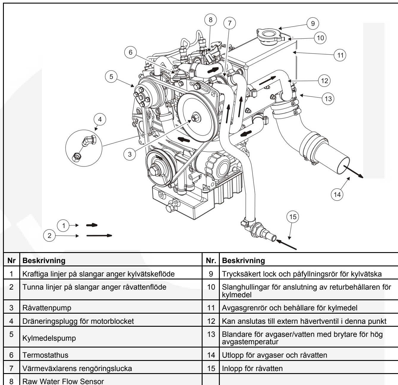
FIGUR 16. KYLSYSTEM
