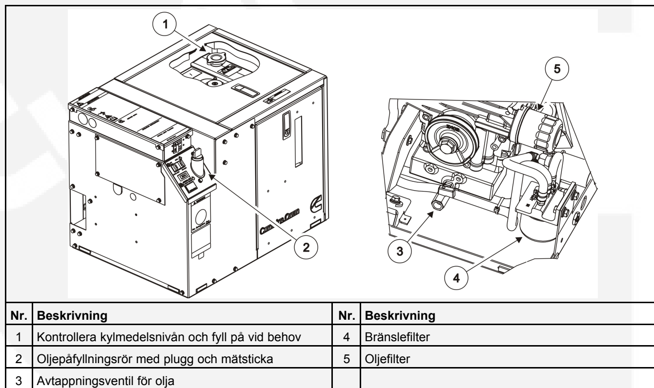
FIGUR 13. SERVICEPUNKTERNAS PLACERING FÖR OLJA OCH BRÄNSLE
