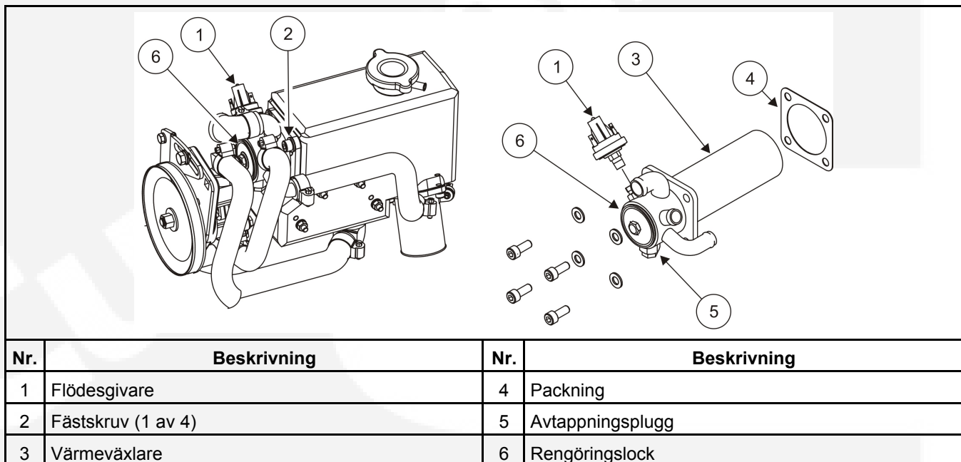
FIGUR 18. VÄRMEVÄXLARE
