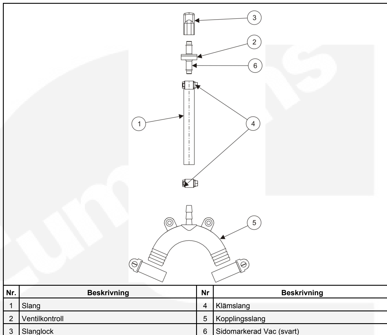
FIGUR 17. HÄVERTVENTIL
