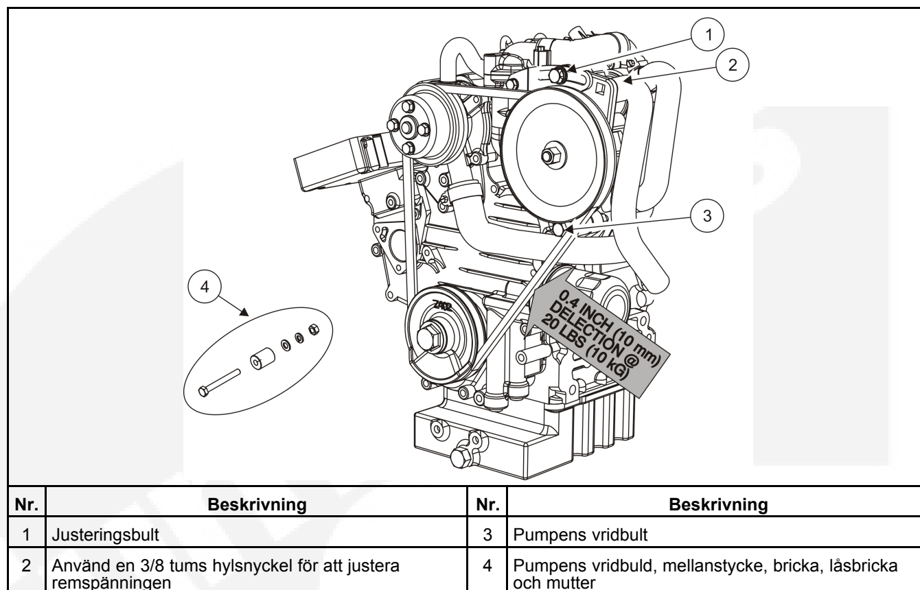
FIGUR 21. JUSTERING AV KILREMMENS SPÄNNING
