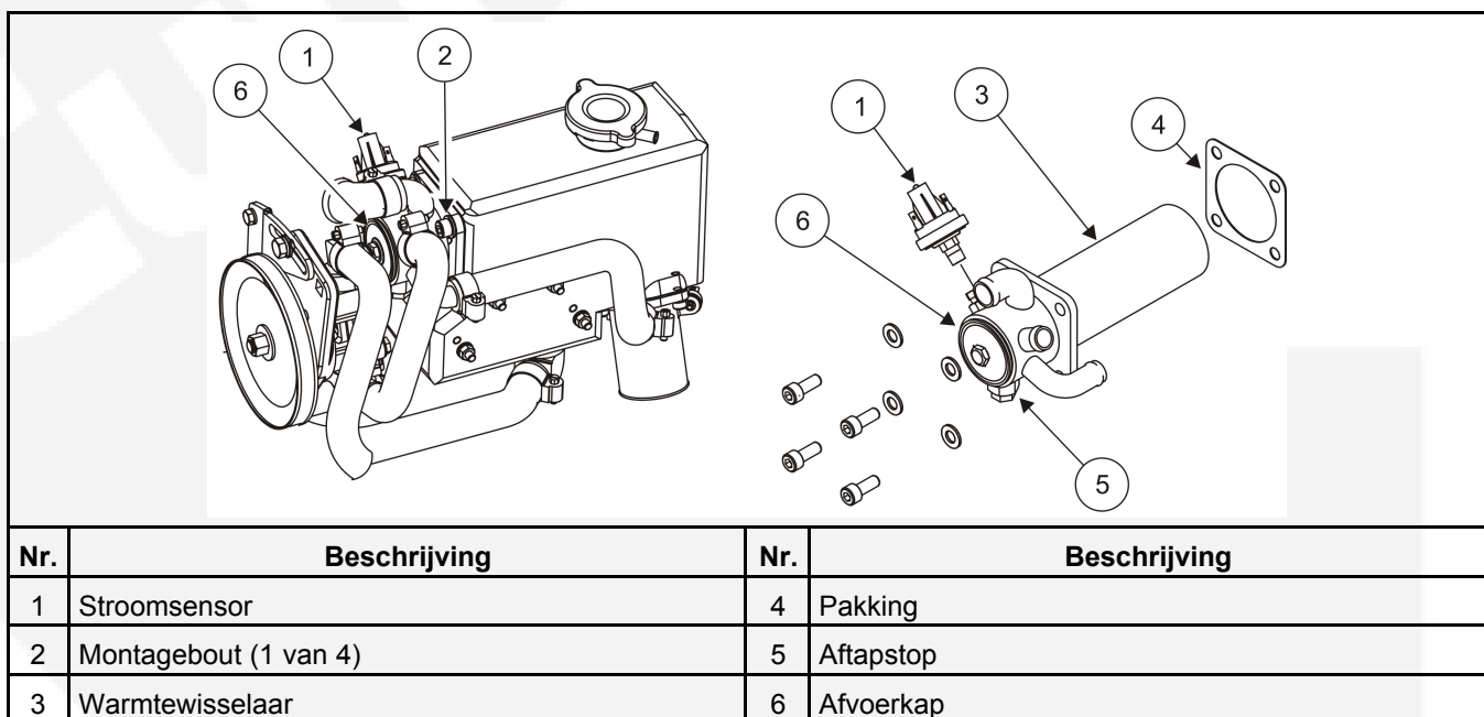
AFBEELDING 18. WARMTEWISSELAAR
