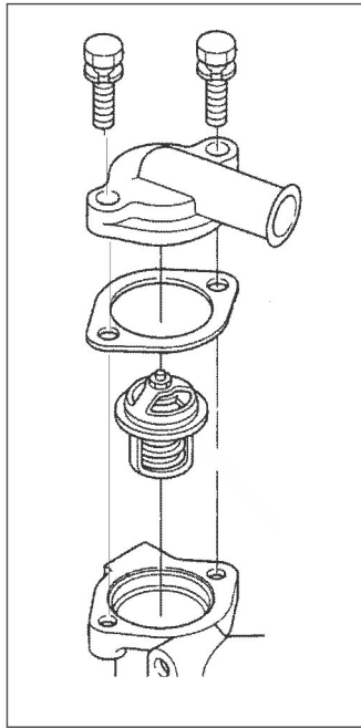
AFBEELDING 19. TYPISCHE THERMOSTAAT MET HUIS
