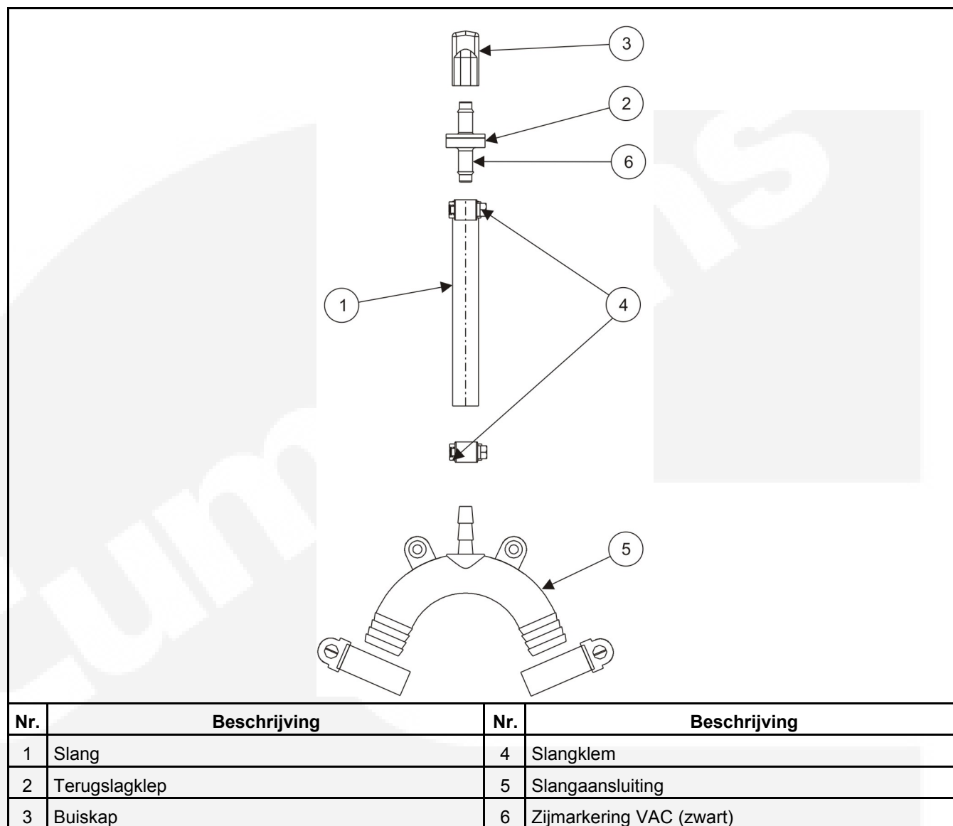
AFBEELDING 17. SIFONONDERBREKING
