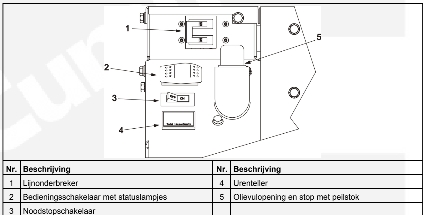
AFBEELDING 4. COMPONENTEN LOKAAL BEDIENINGSPANEEL
