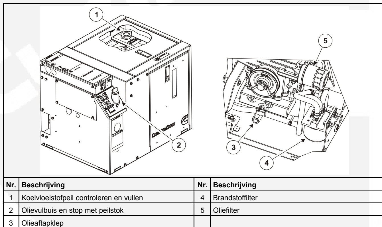
AFBEELDING 13. LOCATIES VAN OLIE- EN BRANDSTOFSERVICEPUNTEN
