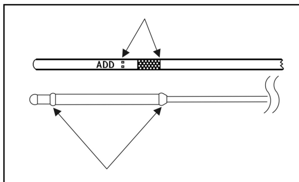
AFBEELDING 14. OLIEPEILSTOKMARKERINGEN BIJVULLEN/VOL
