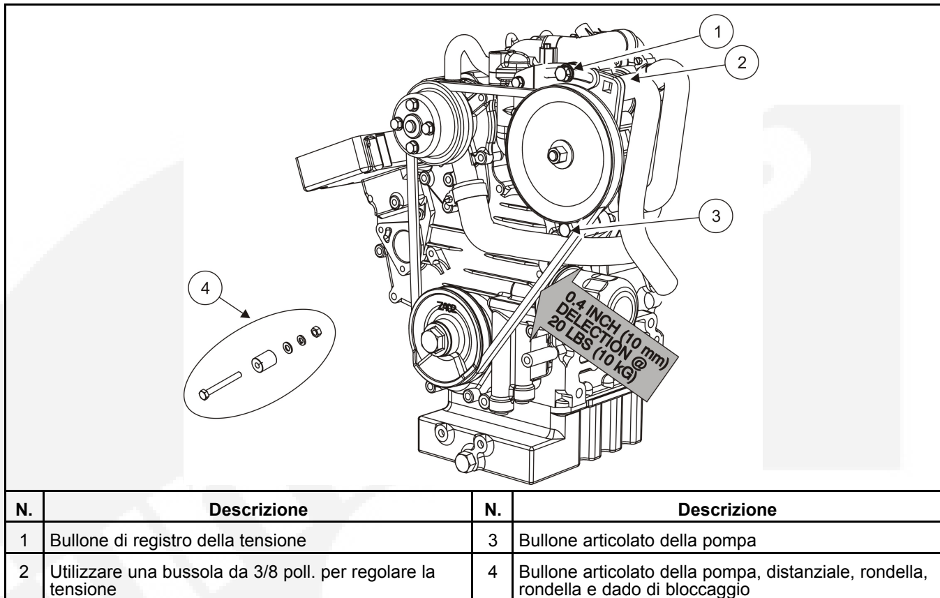
FIGURA 21. REGOLAZIONE DELLA TENSIONE DELLA CINGHIA TRAPEZOIDALE
