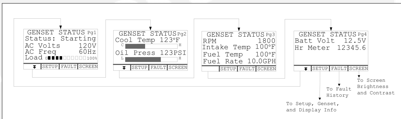
FIGURA 6. SCHERMATE DI STATO DEL GRUPPO GENERATORE
