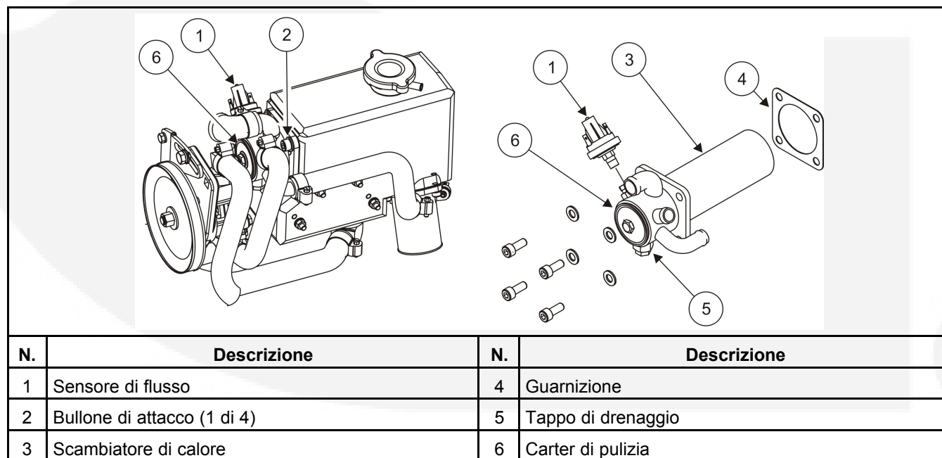
FIGURA 18. SCAMBIATORE DI CALORE
