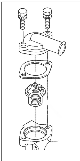
FIGURA 19. TERMOSTATO E ALLOGGIAMENTO DI TIPO COMUNE
