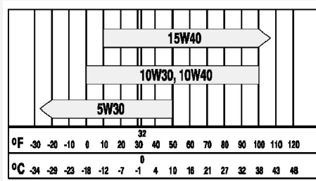
FIGURA 15. VISCOSITÀ DELL'OLIO IN FUNZIONE DELLA TEMPERATURA AMBIENTE
