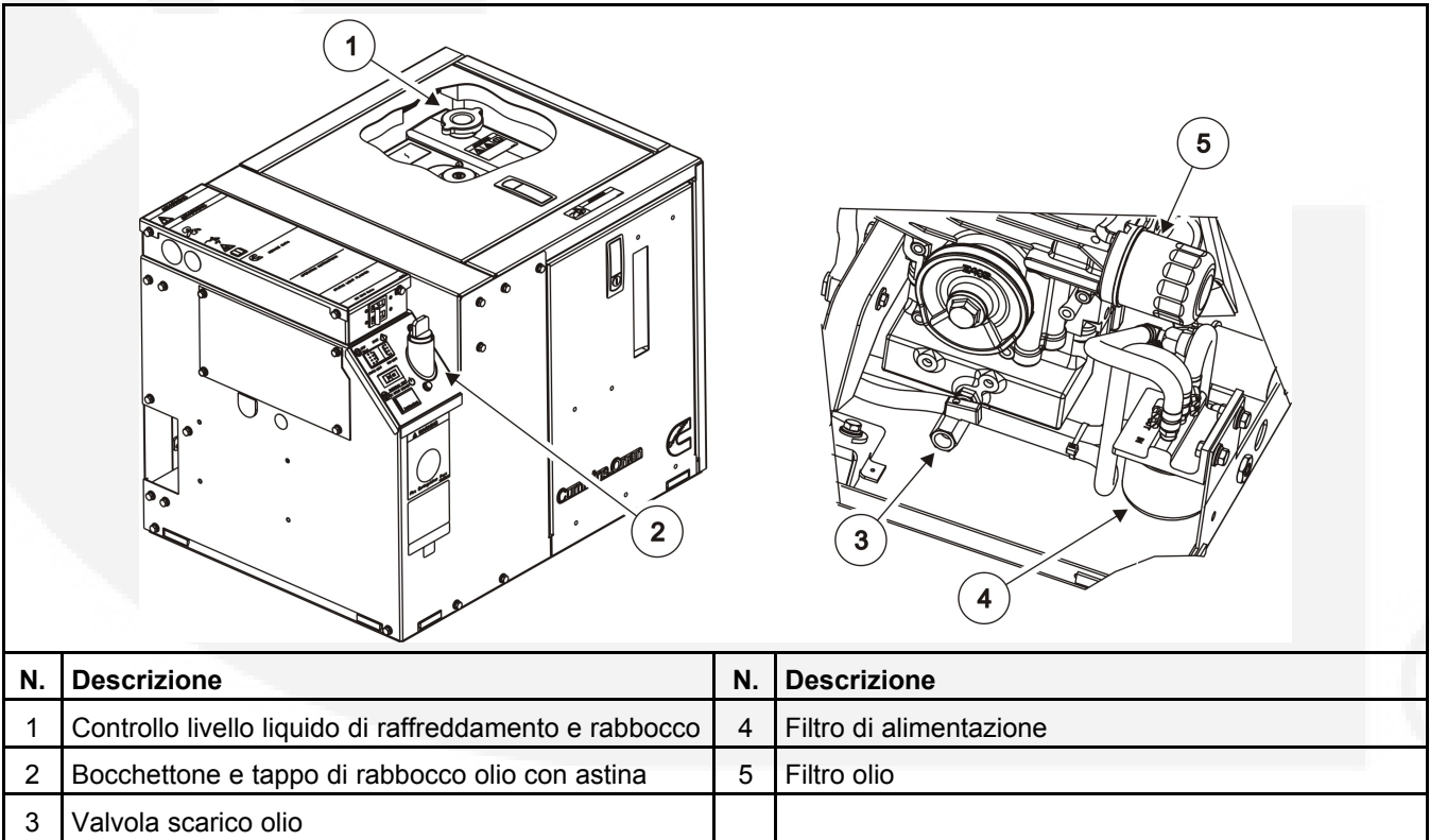
FIGURA 13. POSIZIONE DEI PUNTI DI MANUTENZIONE OLIO E CARBURANTE
