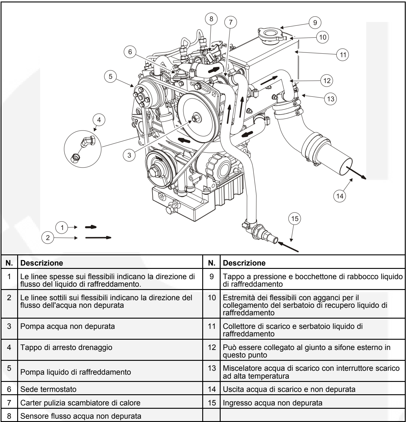
FIGURA 16. IMPIANTO DI RAFFREDDAMENTO
