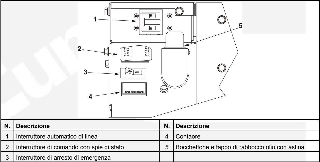
FIGURA 4. COMPONENTI QUADRO DI COMANDO LOCALE
