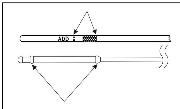
FIGURA 14. TACCHE ADD/FULL DELL'ASTINA OLIO
