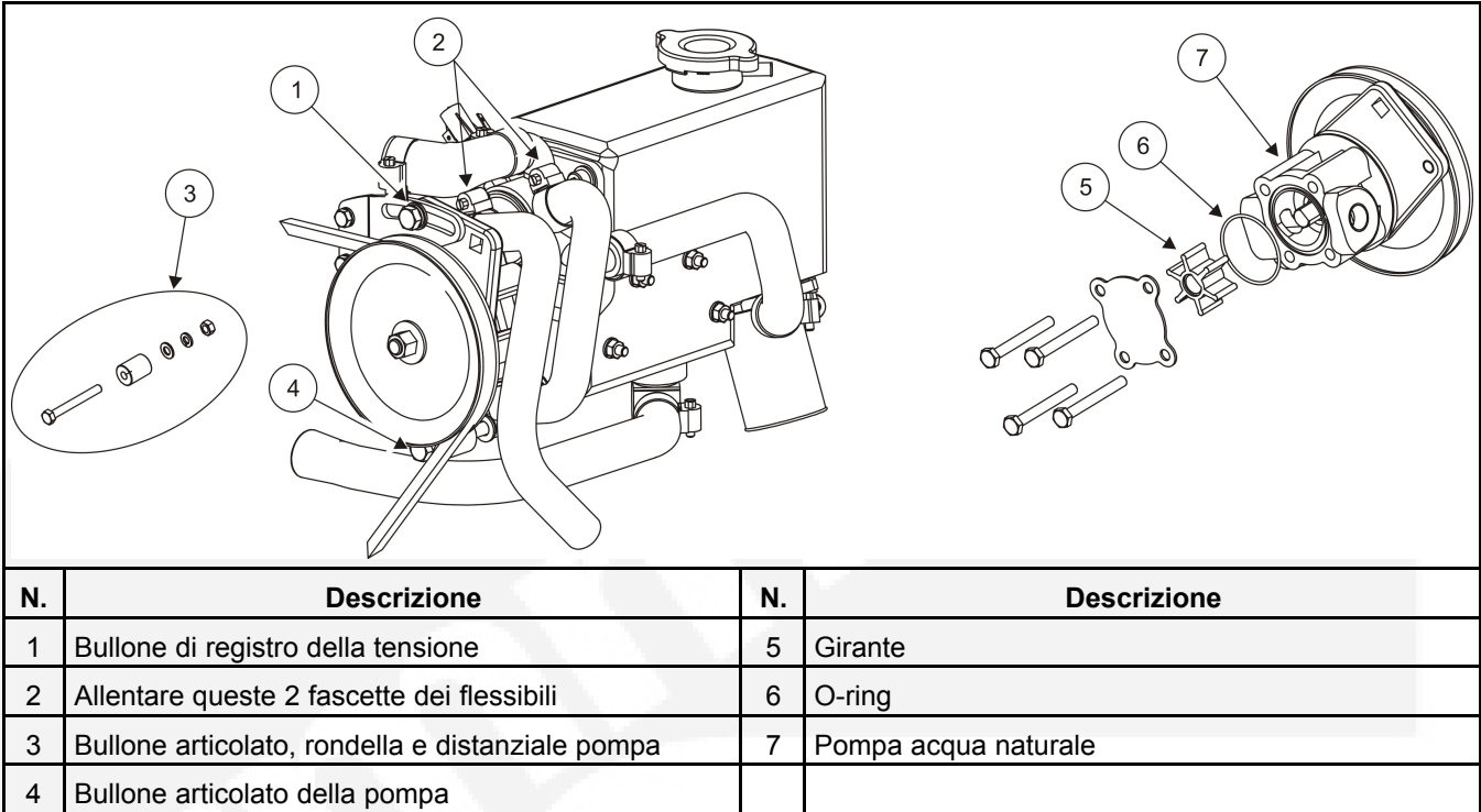
FIGURA 20. SMONTAGGIO POMPA ACQUA NATURALE
