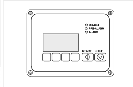
FIGURA 5. PANTALLA DIGITAL CUMMINS ONAN
