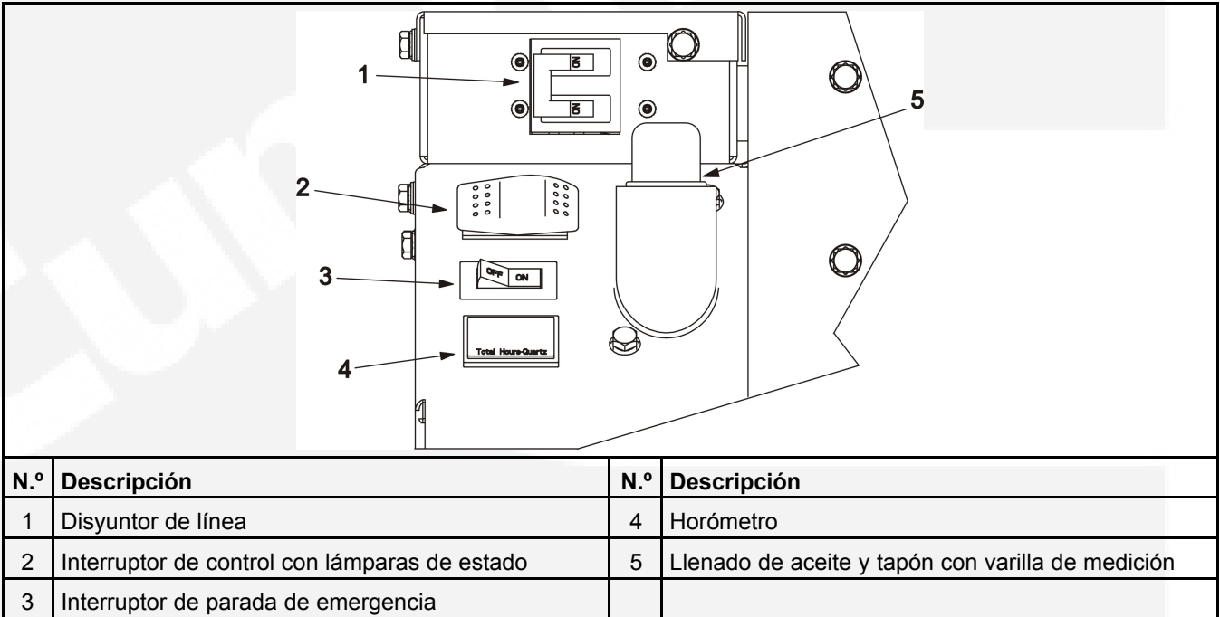
FIGURA 4. COMPONENTES DEL TABLERO DE CONTROL LOCAL
