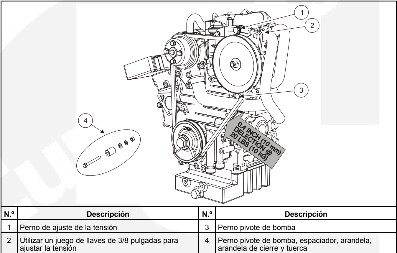
FIGURA 21. AJUSTE DE TENSIÓN DE CORREA TRAPEZOIDAL
