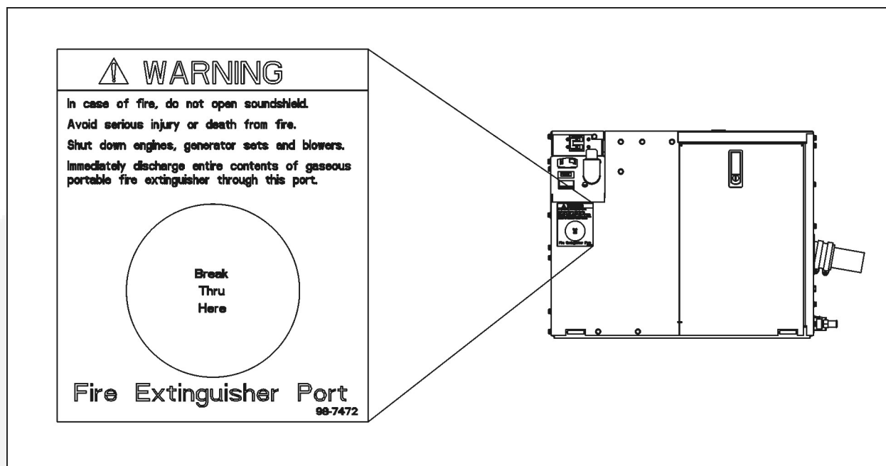
FIGURA 12. UBICACIÓN DE LA ETIQUETA DEL PUERTO DE EXTINCIÓN DE INCENDIOS
