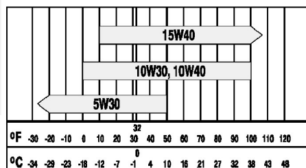
FIGURA 15. VISCOSIDAD DEL ACEITE FRENTE A TEMPERATURA AMBIENTE
