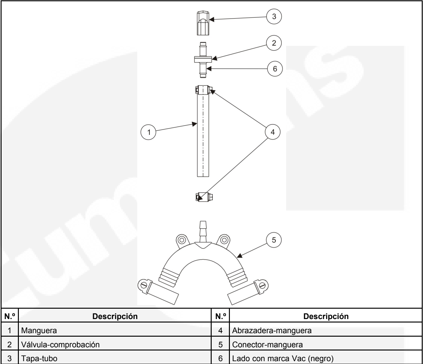
FIGURA 17. RESPIRADERO DE SIFÓN
