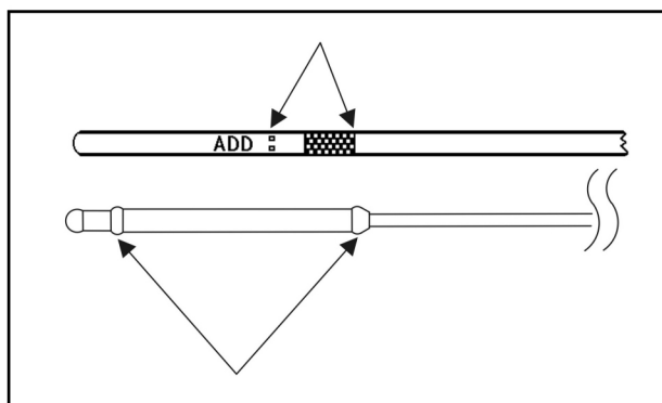
FIGURA 14. MARCAS ADD (AÑADIR)/FULL (LLENO) DE LA VARILLA DE MEDICIÓN DEL NIVEL DE ACEITE
