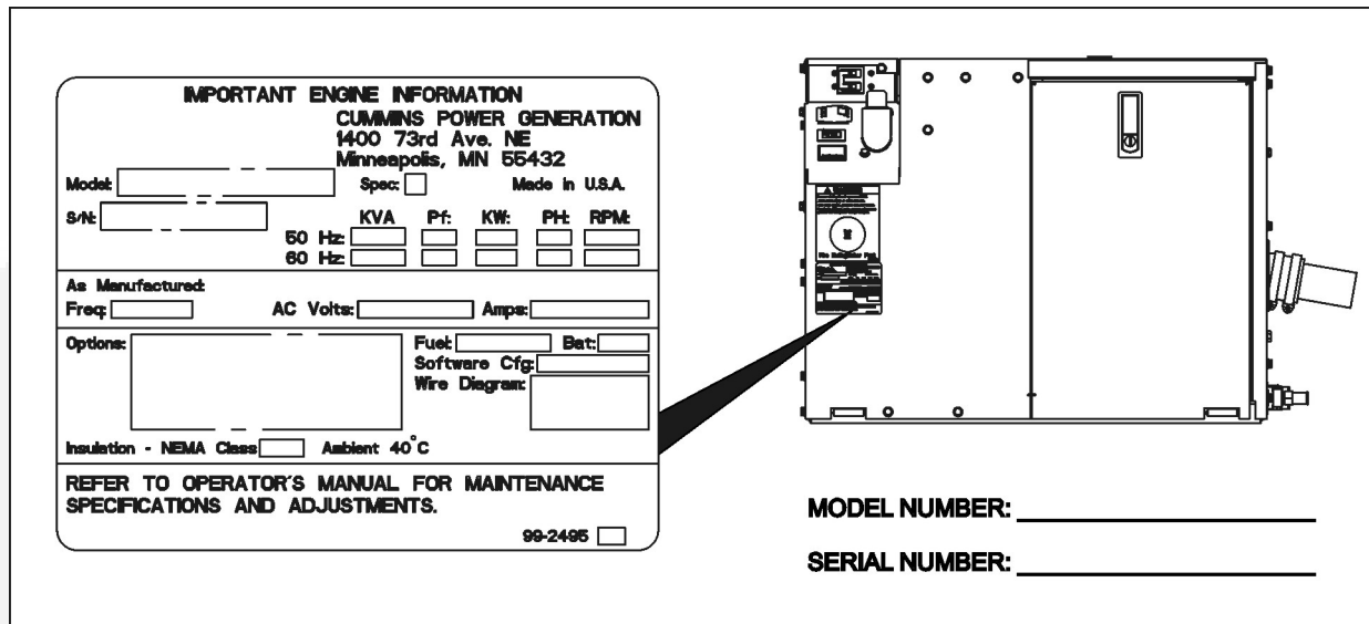
FIGURA 2. UBICACIÓN DE LA CHAPA DE IDENTIFICACIÓN
