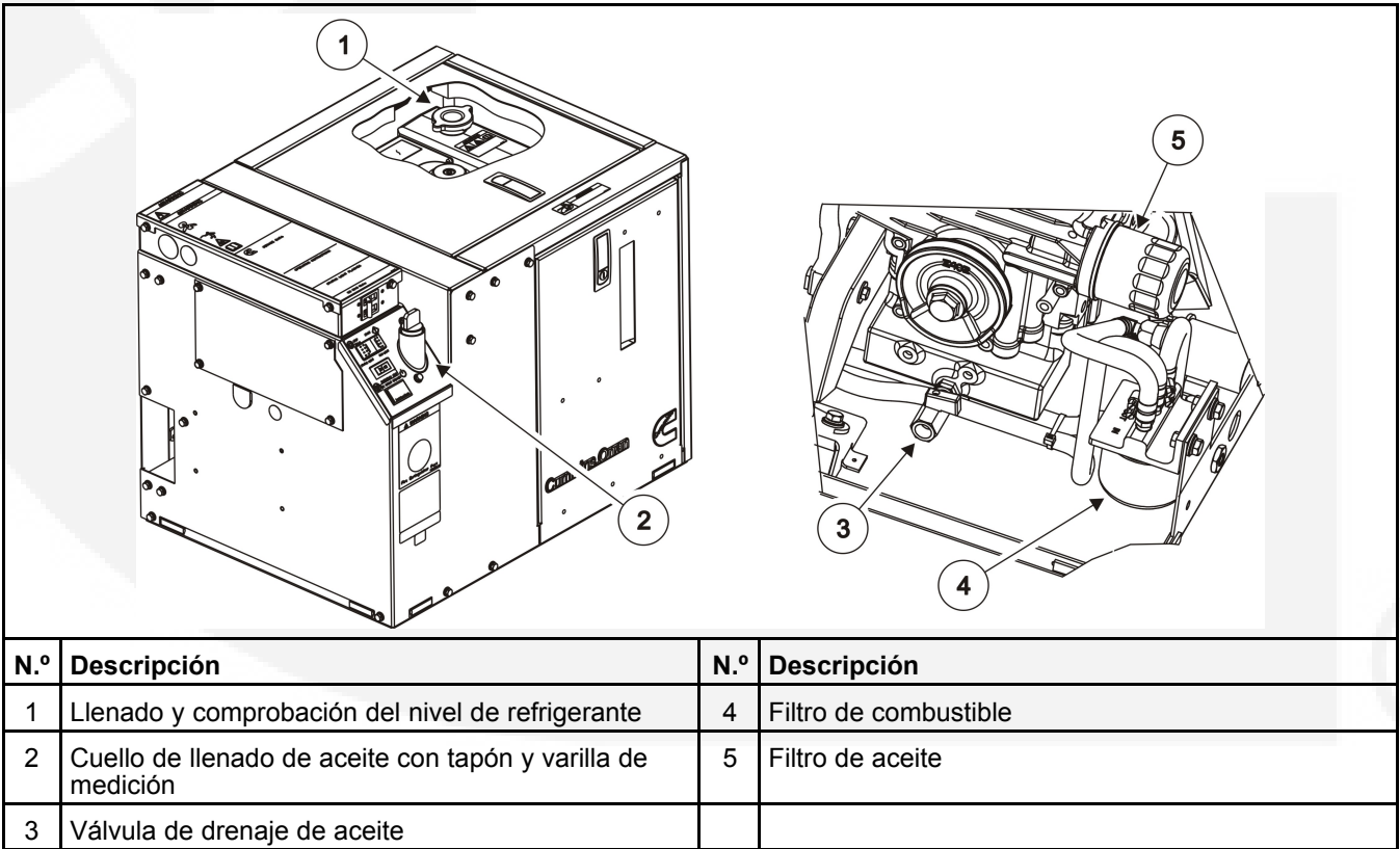
FIGURA 13. UBICACIONES DE LOS PUNTOS DE SERVICIO DEL ACEITE Y EL COMBUSTIBLE
